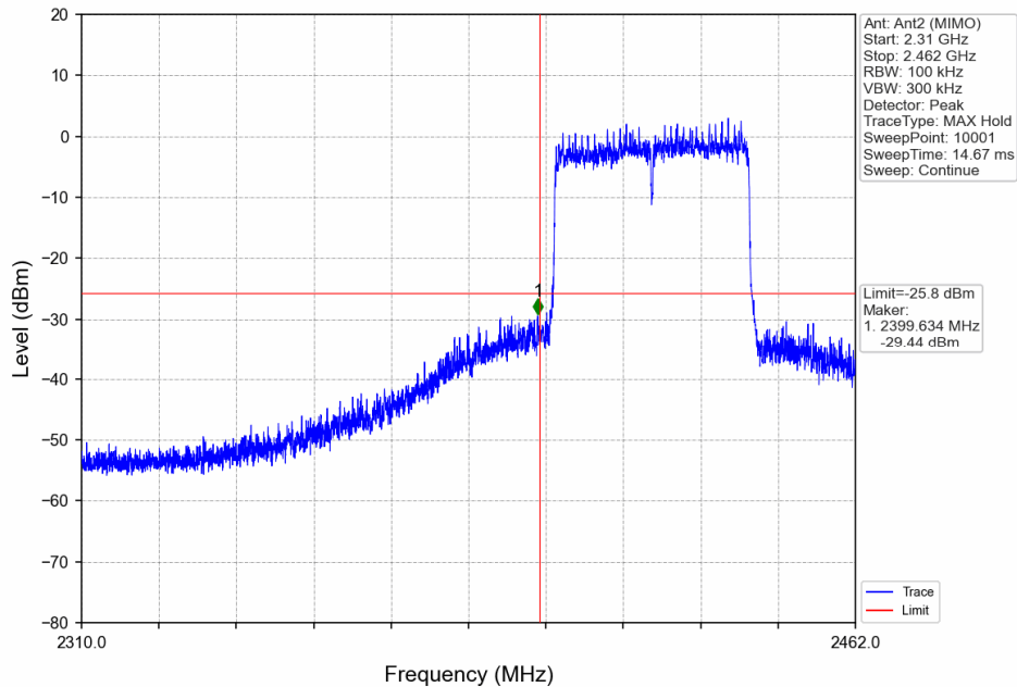
802.11ax(HEW40)_LCH_2422MHz_RU484_Left_Ant2 (MIMO)_NTNV
