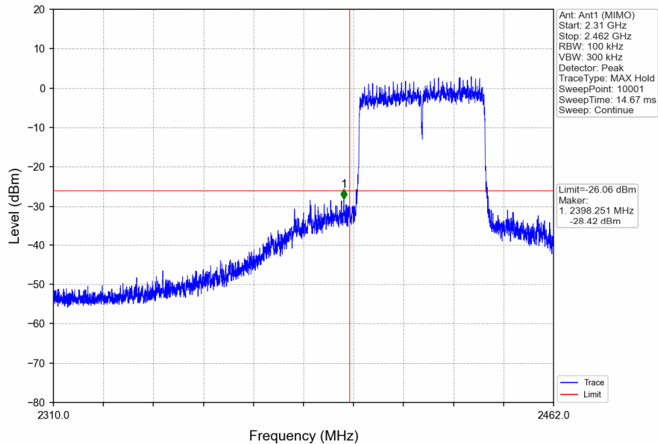
802.11ax(HEW40)_LCH_2422MHz_RU484_Left_Ant1 (MIMO)_NTNV
