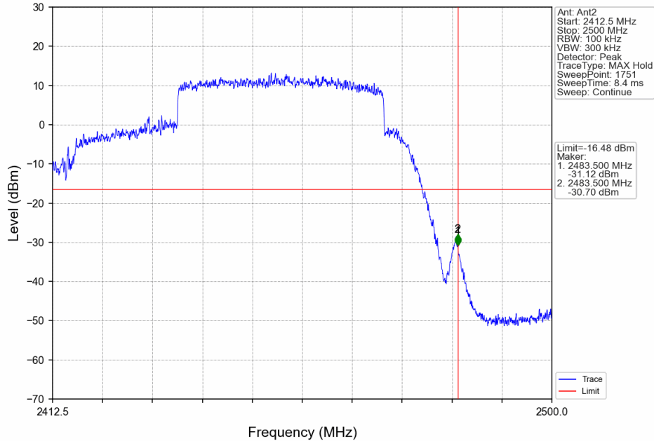
40M_HCH_2452.5MHz_Ant2_NTNV
