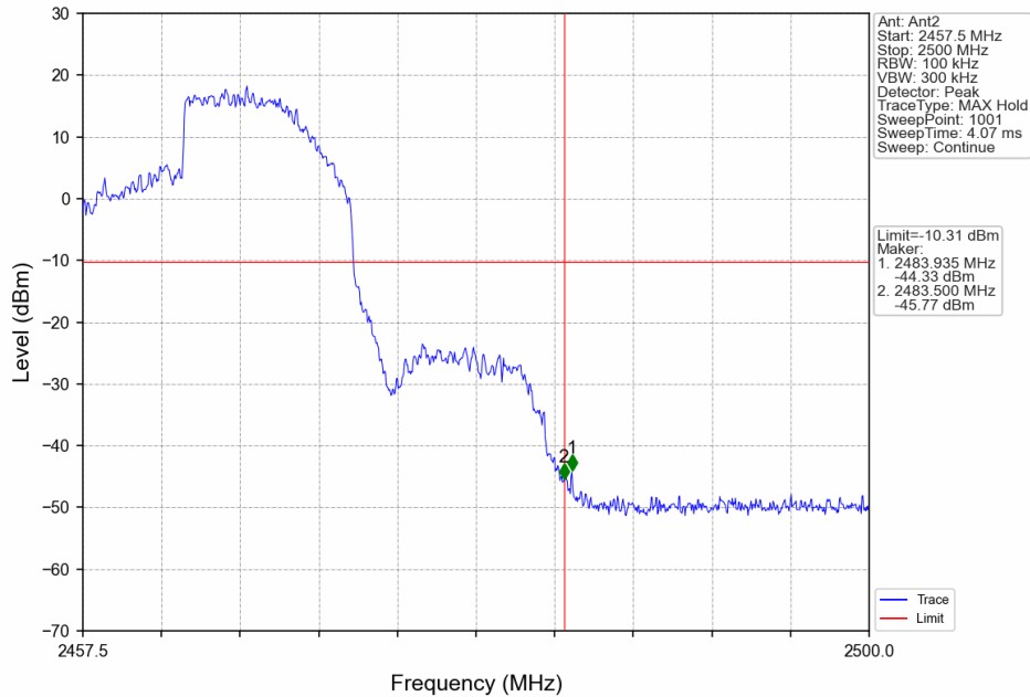
10M_HCH_2467.5MHz_Ant2_NTNV
