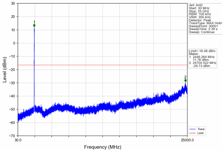
40M_HCH_2452.5MHz_Ant2_NTNV
