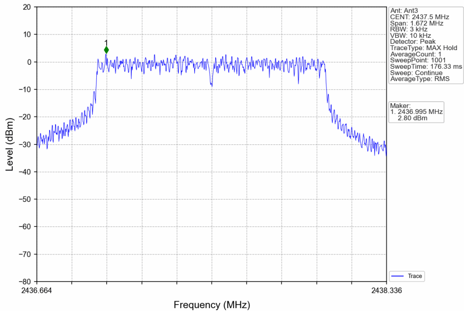
1.4M_MCH_2437.5MHz_Ant3_NTNV
