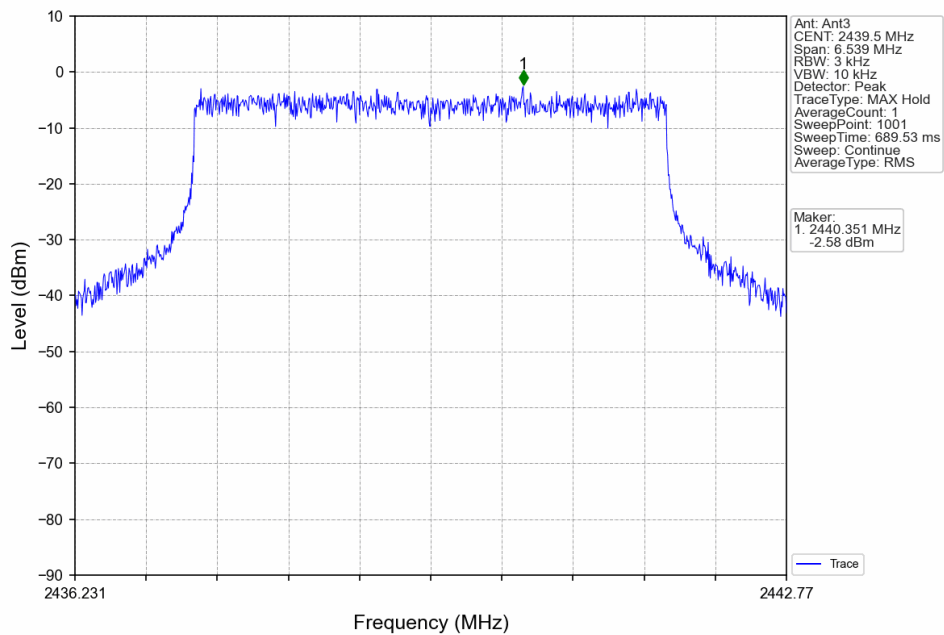
5M_MCH_2439.5MHz_Ant3_NTNV
