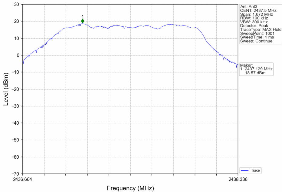
1.4M_MCH_2437.5MHz_Ant3_NTNV
