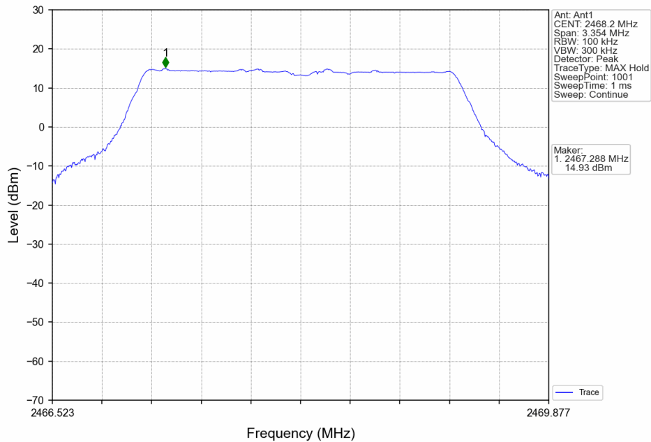
3M_HCH_2468.2MHz_Ant1_NTNV
