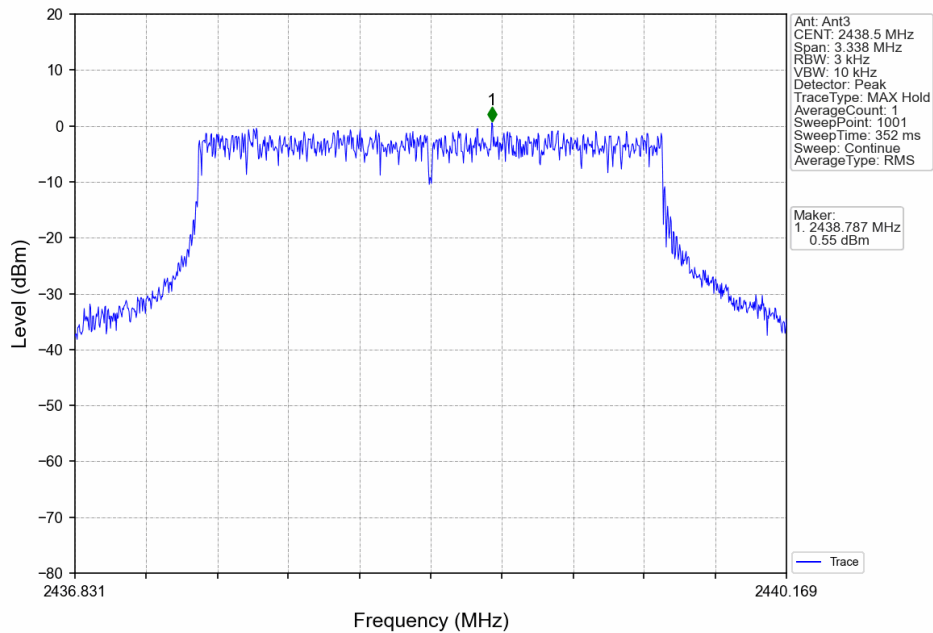
3M_MCH_2438.5MHz_Ant3_NTNV
