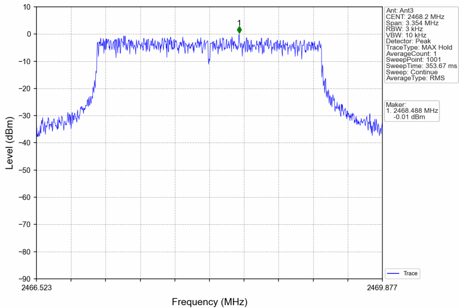
3M_HCH_2468.2MHz_Ant3_NTNV
