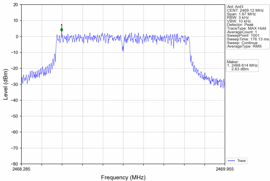
1.4M_HCH_2469.12MHz_Ant3_NTNV
