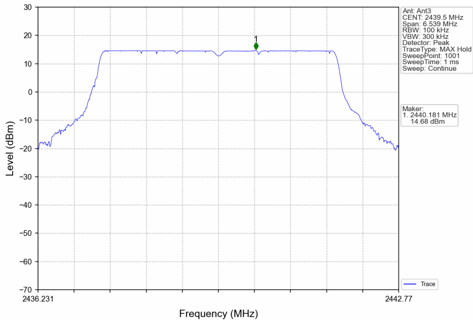
5M_MCH_2439.5MHz_Ant3_NTNV
