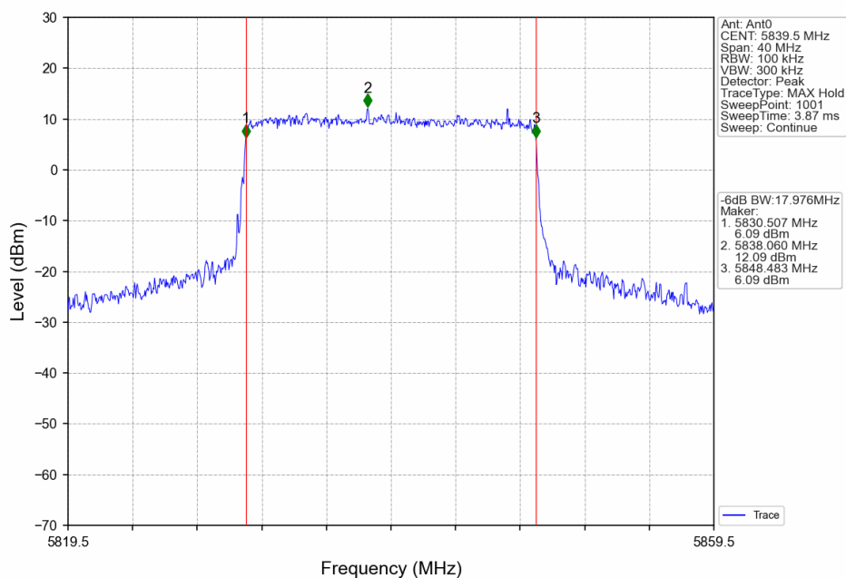
20M_HCH_5839.5MHz_Ant0_NTNV
