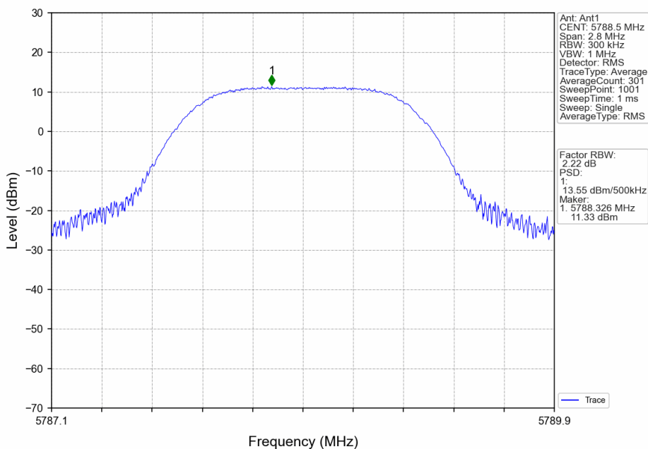
1.4M_MCH_5788.5MHz_MIMO_NTNV
