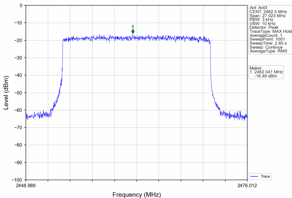
20M_HCH_2462.5MHz_Ant3_NTNV
