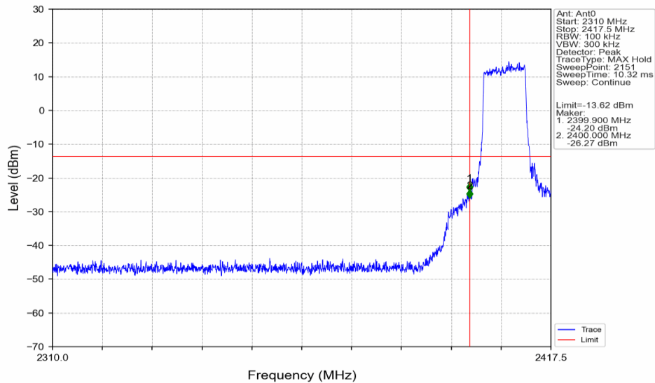
10M_LCH_2407.5MHz_Ant0_NTNV
