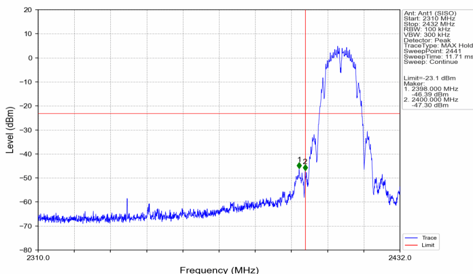
802.11b_LCH_2412MHz_Ant1 (SISO)_NTNV
