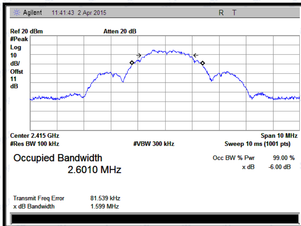
(Plot A: Channel 0: 2415MHz)
