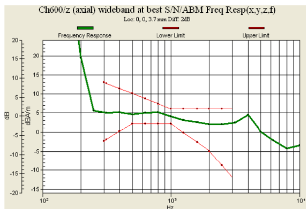
Fig 7.5 CDMA2000 BC1 Ch600
