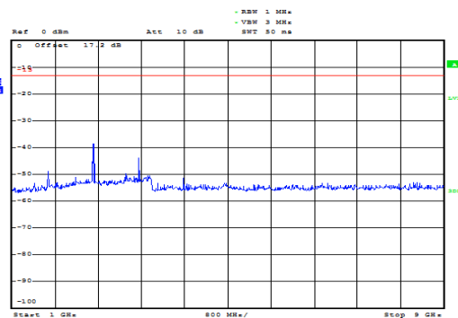
GSM 850 CH-Middle 1GHz ~ 9GHz
