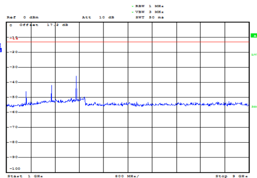
GSM 850 CH-Low 1GHz ~ 9GHz
