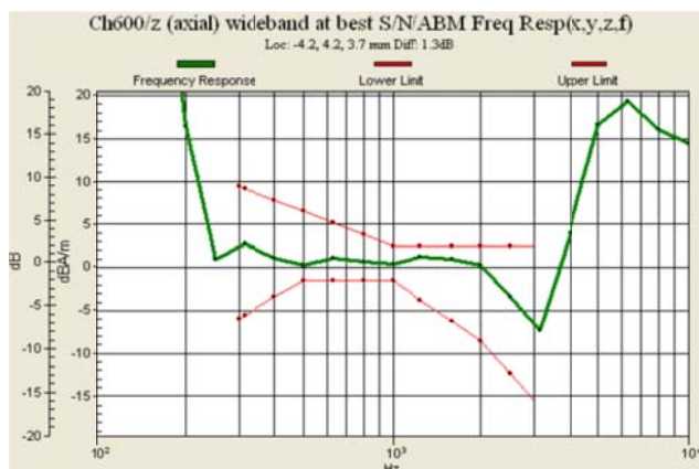
Fig 7.5 CDMA2000 BC1 Ch600
