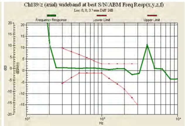
Fig 7.2 GSM850 Ch189
