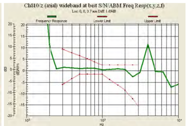
Fig 7.6 GSM1900 Ch810
