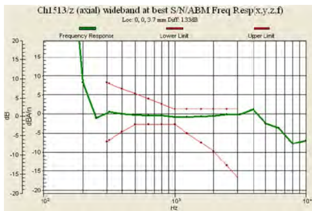
Fig. 7.11 WCDMA Band IV Ch1513
