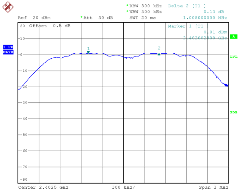
\pi/4 -DQPSK Low Mode
