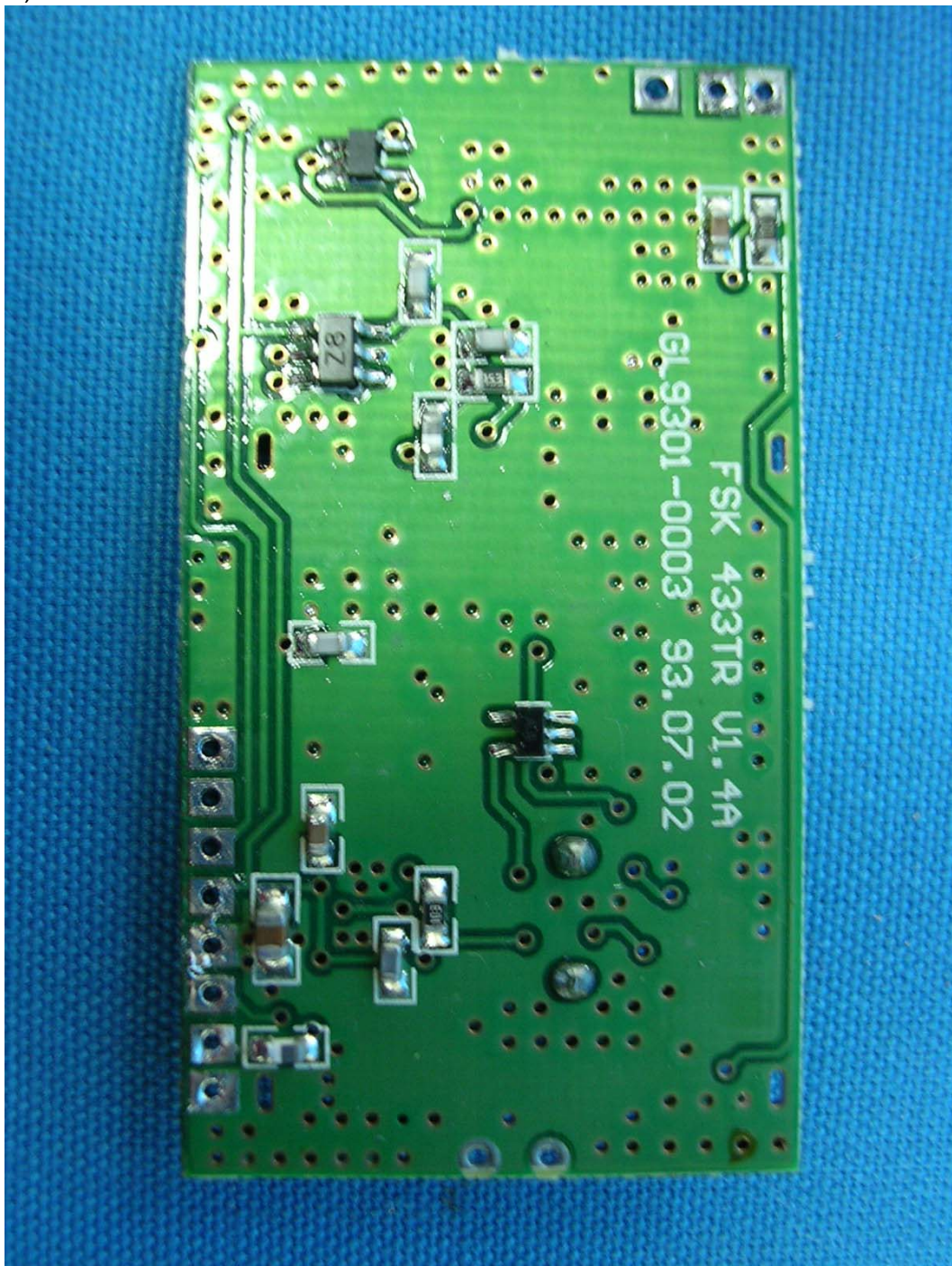
(21) EUT Photo
