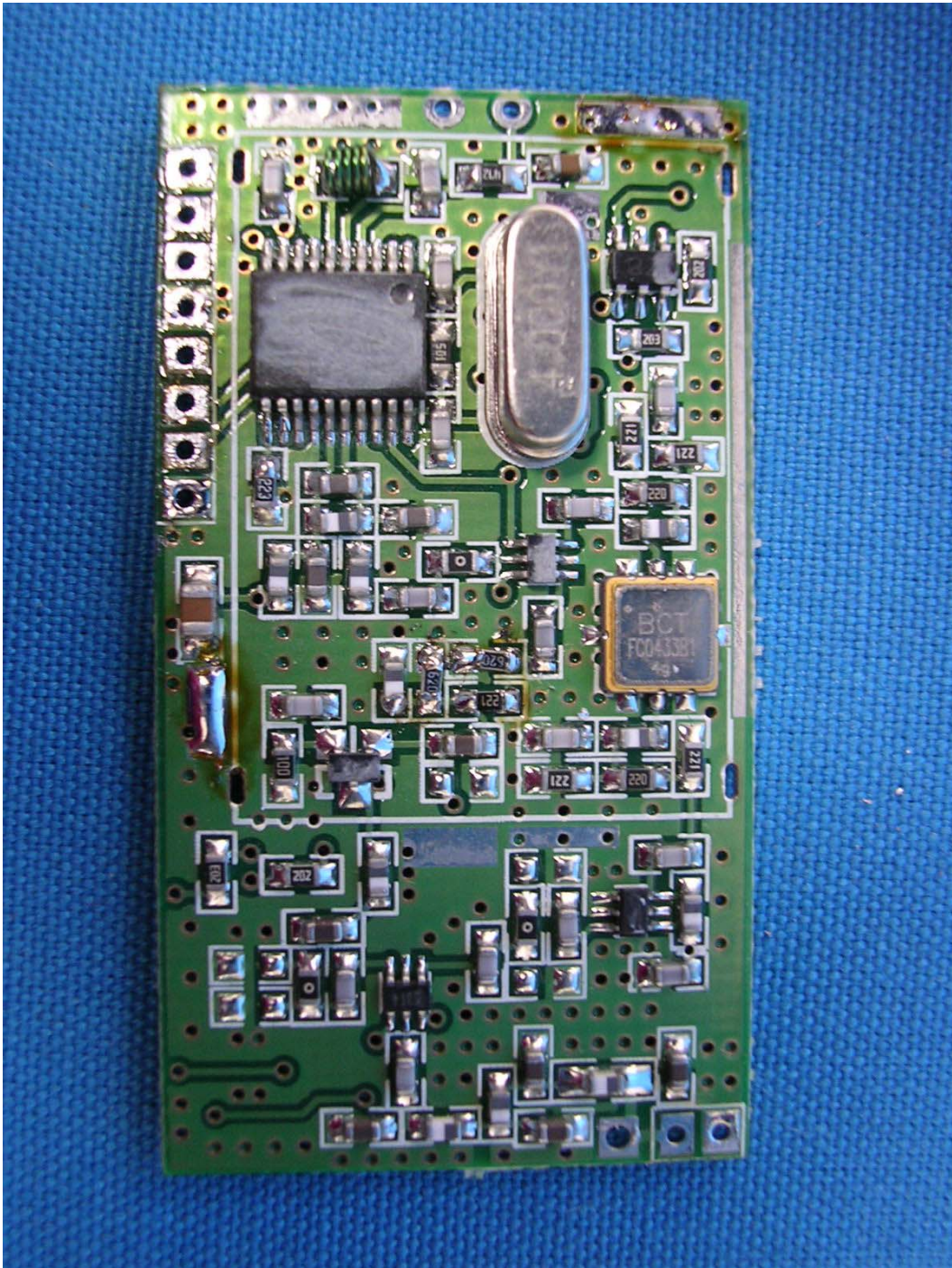
(20) EUT Photo
