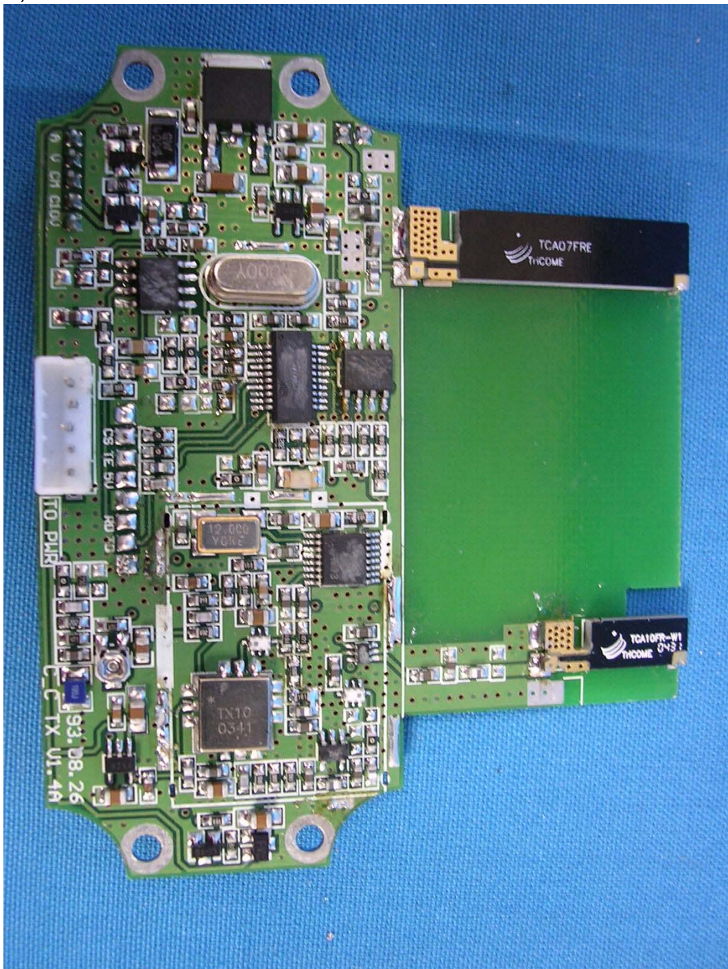
(17) EUT Photo
