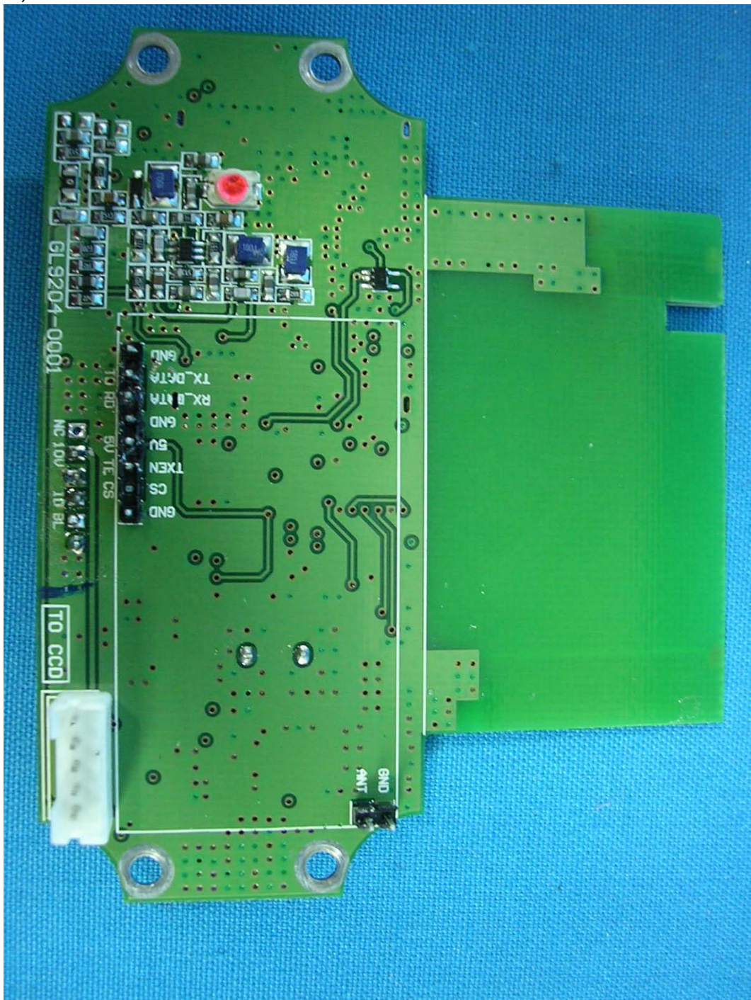
(18) EUT Photo
