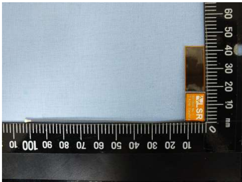
Antenna: FlexPIFA
