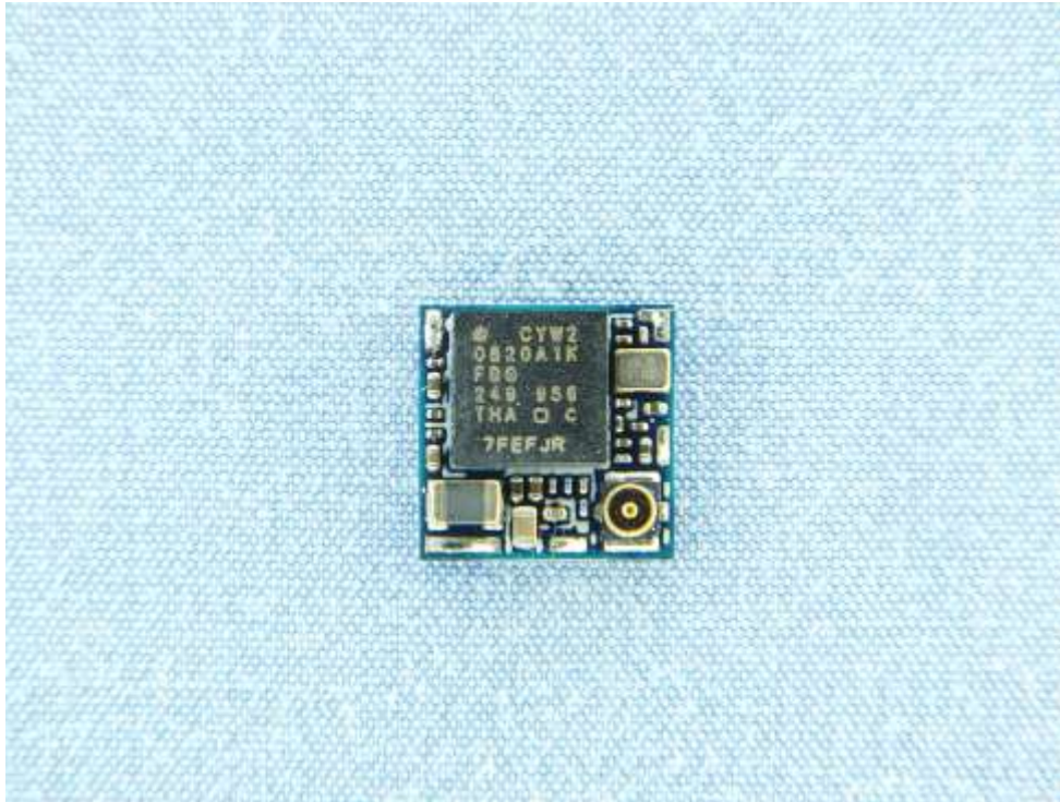
Antenna: mFlexPIFA
