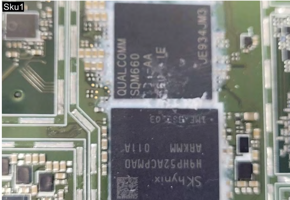
EUT Photo (36)
