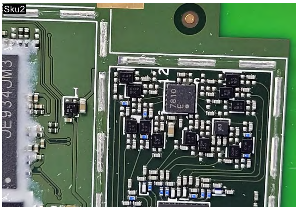
EUT Photo (112)
