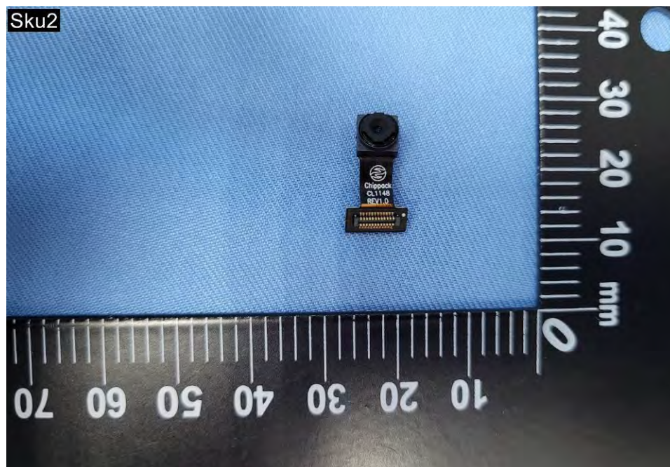
EUT Photo (100)
