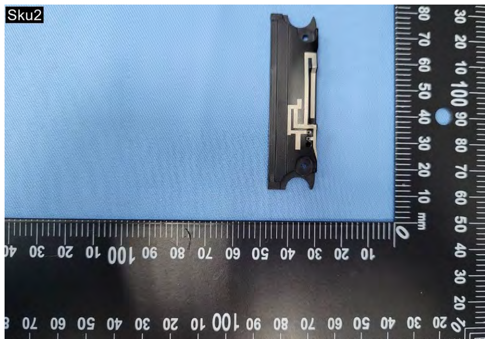
EUT Photo (74)
