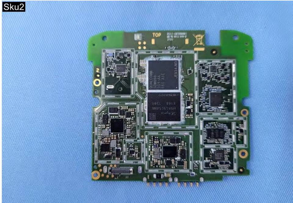
EUT Photo (106)
