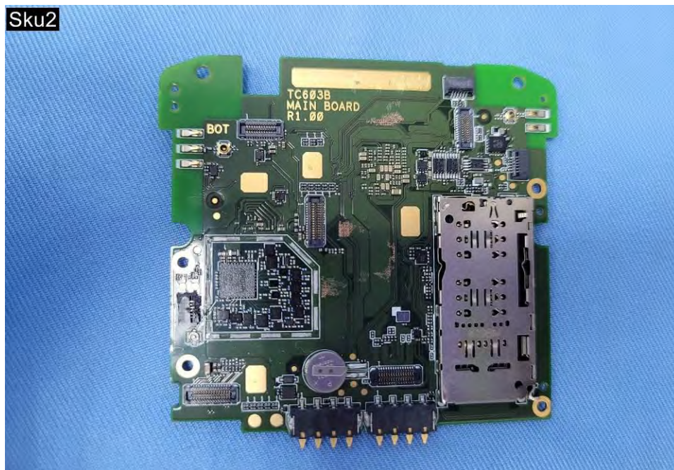
EUT Photo (102)
