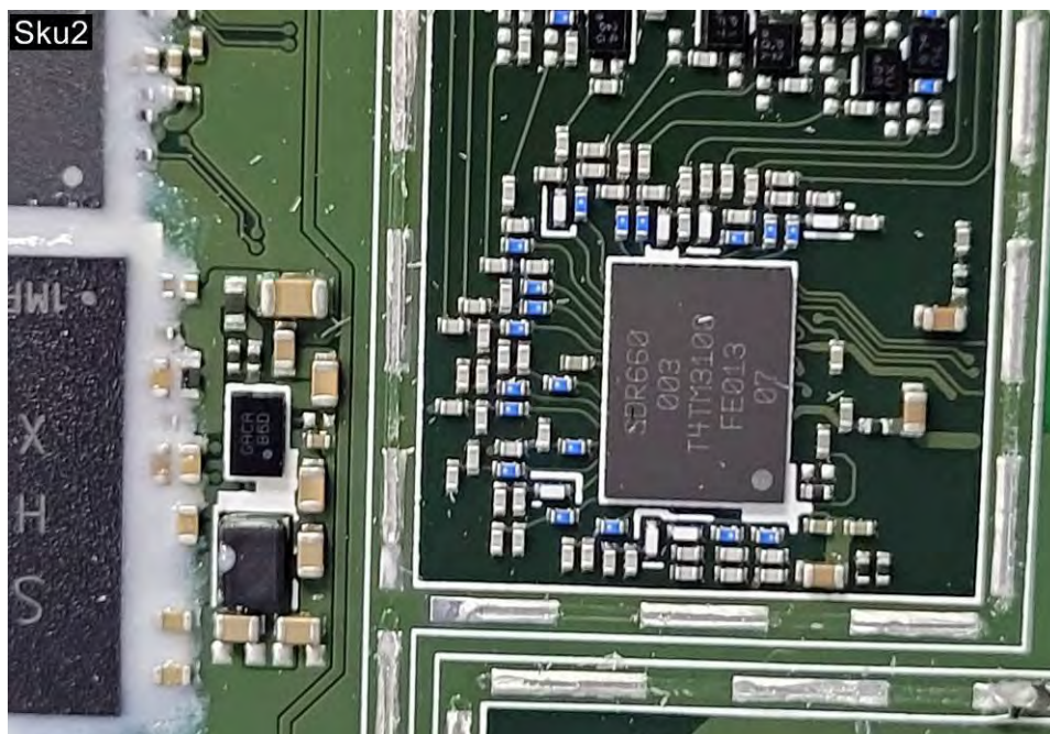
EUT Photo (110)
