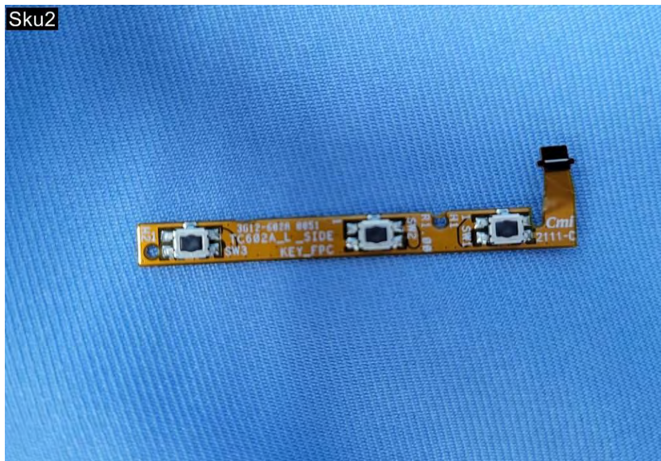
EUT Photo (124)
