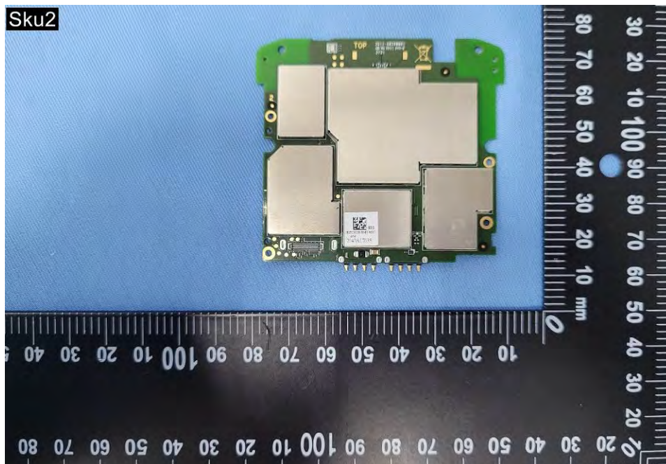
EUT Photo (104)
