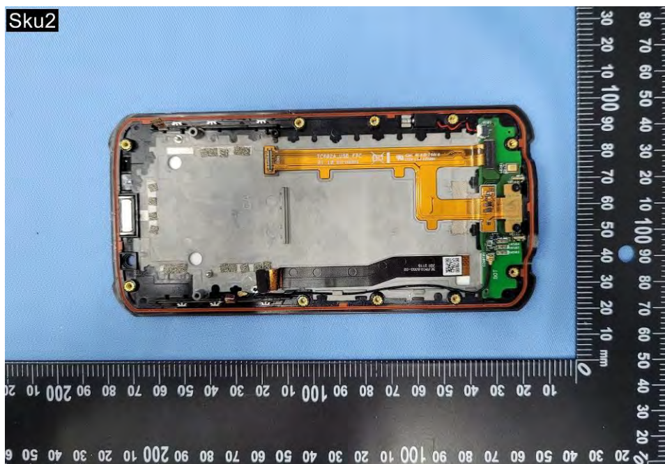
EUT Photo (112)
