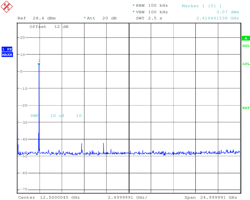
Plot 4: (OFDM)
