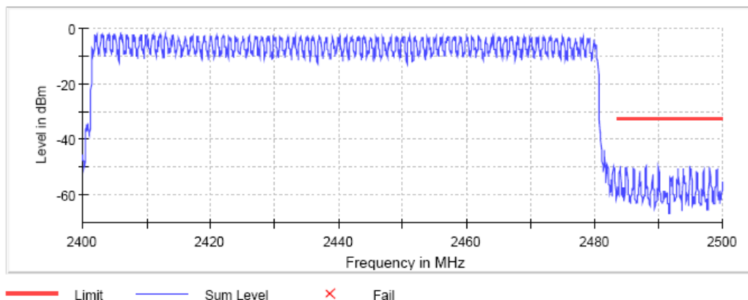
Band Edge
