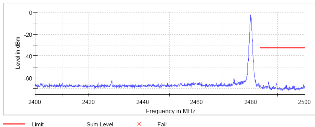
Band Edge
