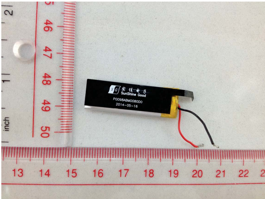
BATTERY(1)
