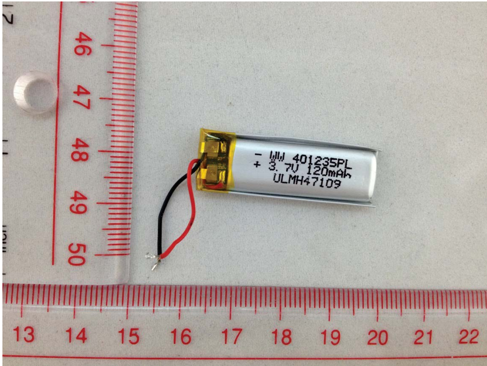
BATTERY(2)
