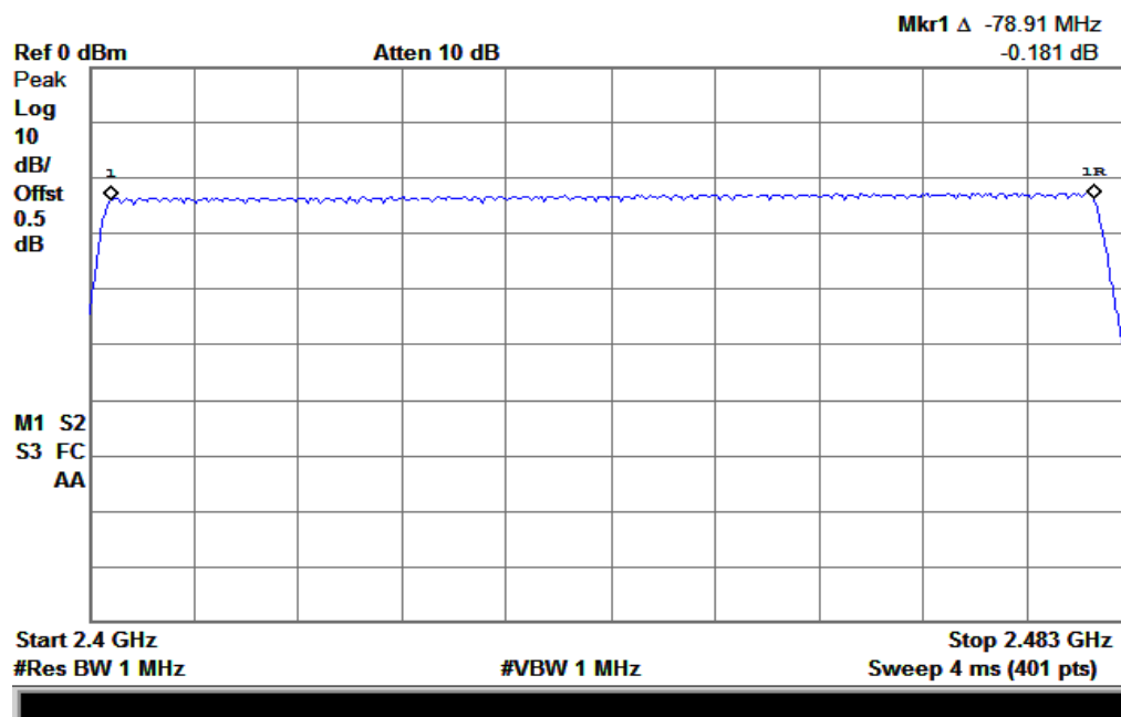
(Plot B: \pi/4 -DQPSK)
