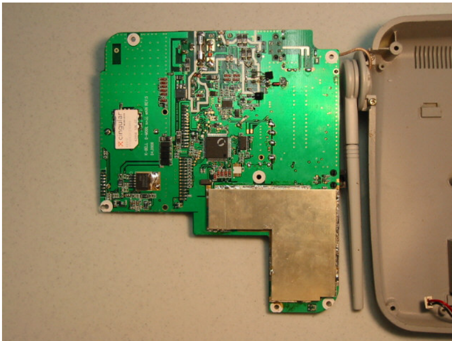
Dmode PCB Base Bottom
