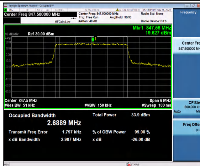
Band5-3MHz-QPSK-20635-15RB#0-2.6889
