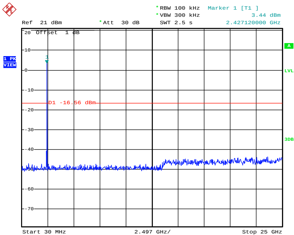
(Plot 4.6.1 A: Channel 1: 2412MHz @ 802.11b)
