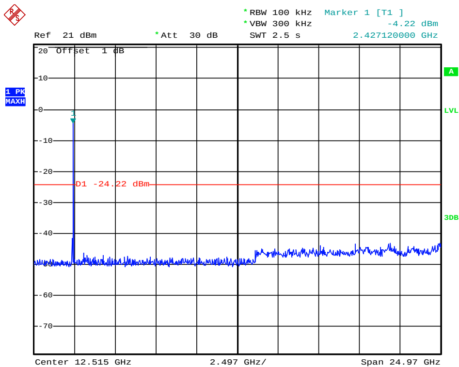
(Plot 4.6.2 A: Channel 1: 2412MHz @ 802.11g)
