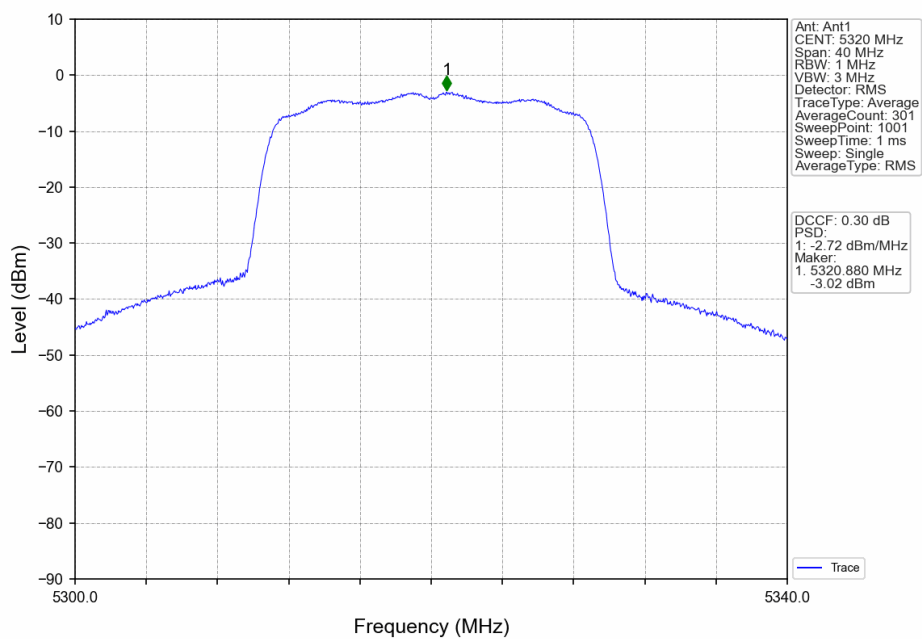
802.11n(HT20)_HCH_5320MHz_Ant1_NTNV
