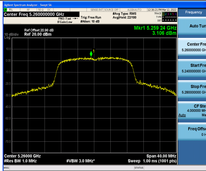
11AC20MIMO_Ant2_5260
