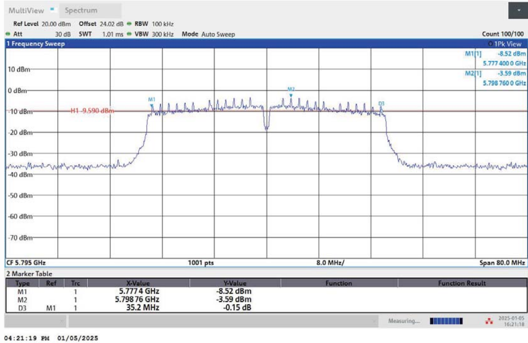
11N40MIMO-Ant1-5795-PASS
