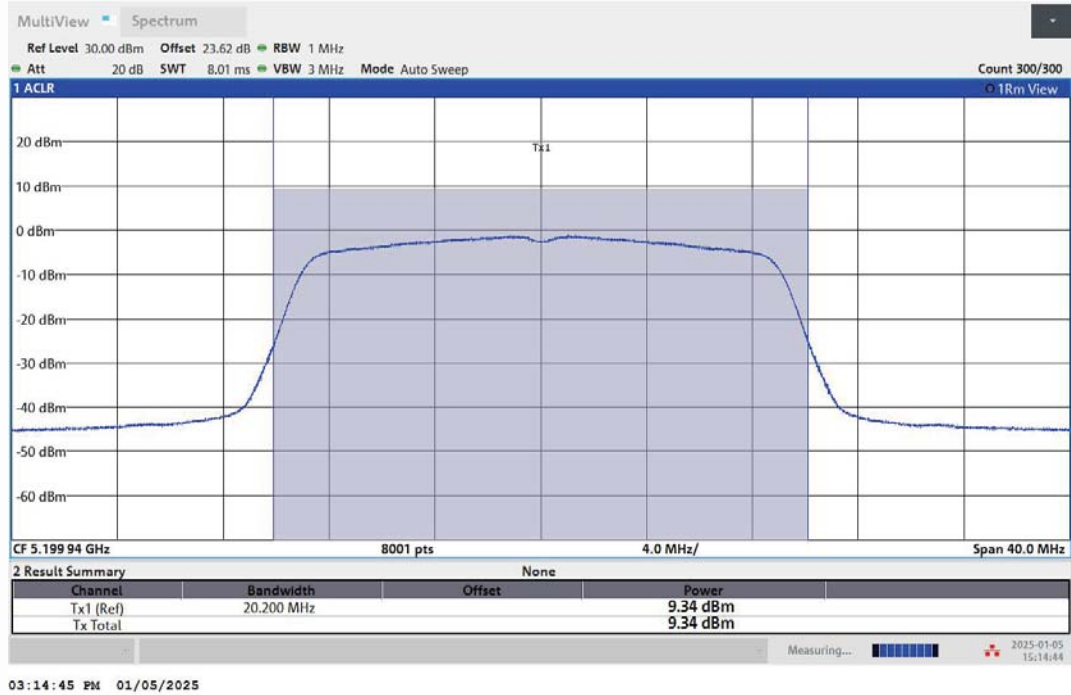
11N20MIMO-Ant1-5200-PASS
