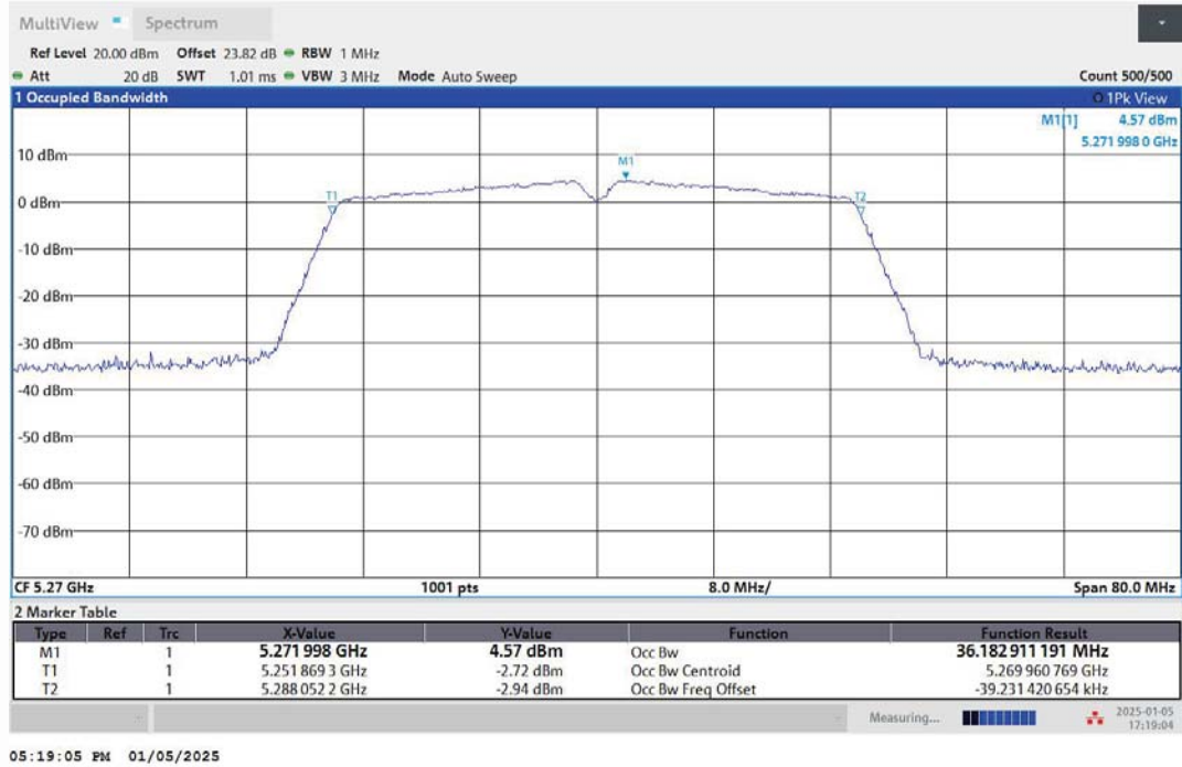
11AC40MIMO-Ant1-5270
