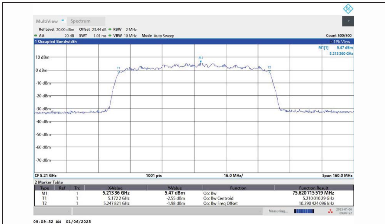
11AC80MIMO-Ant1-5210
