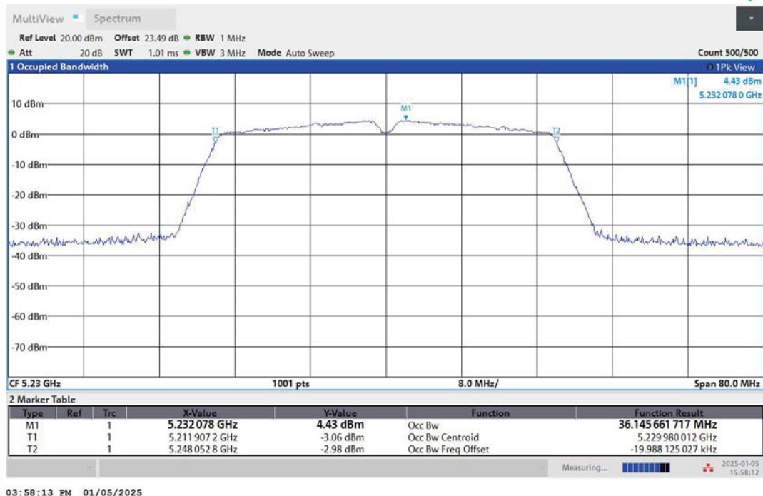
11N40MIMO-Ant1-5230
