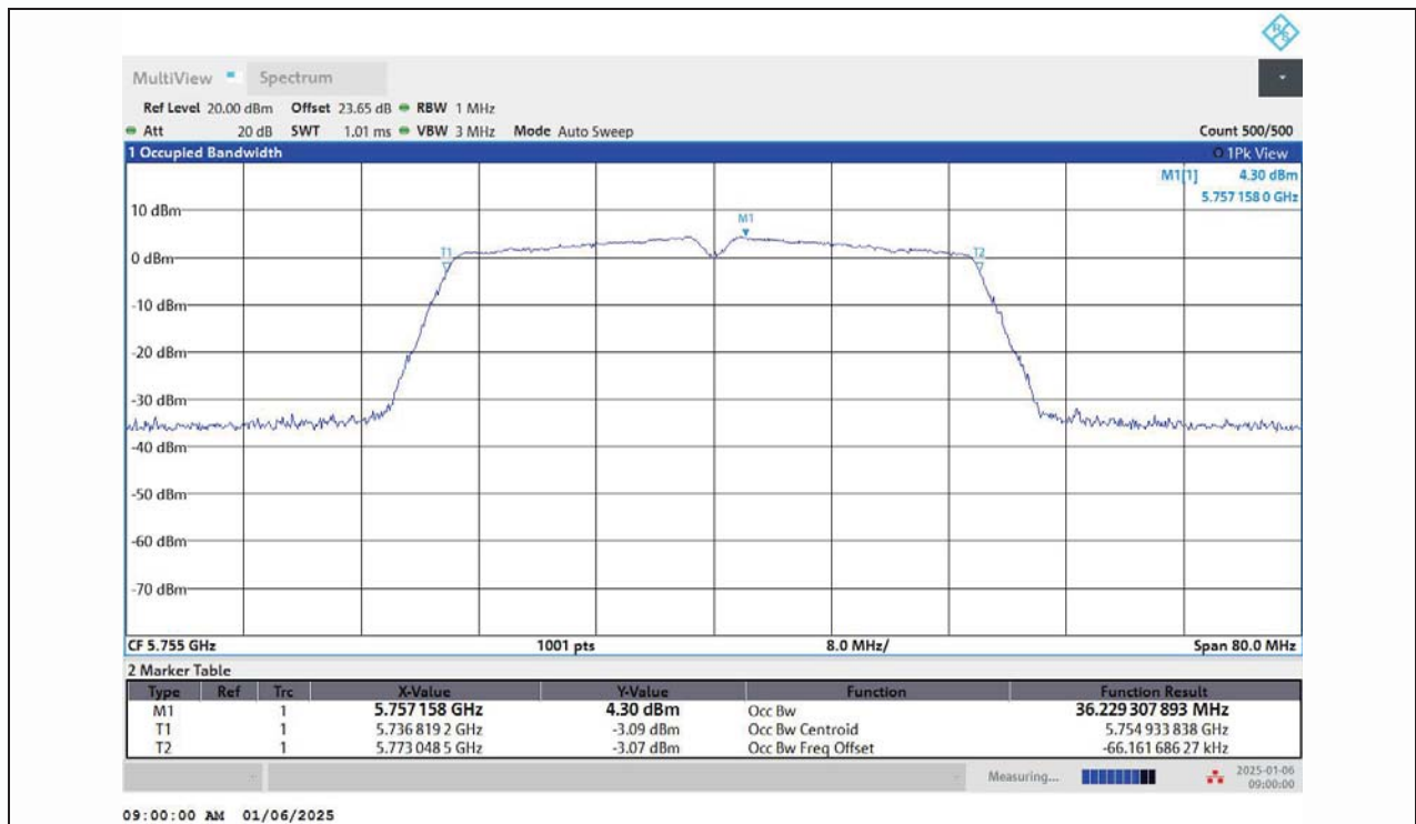
11AC40MIMO-Ant1-5755
