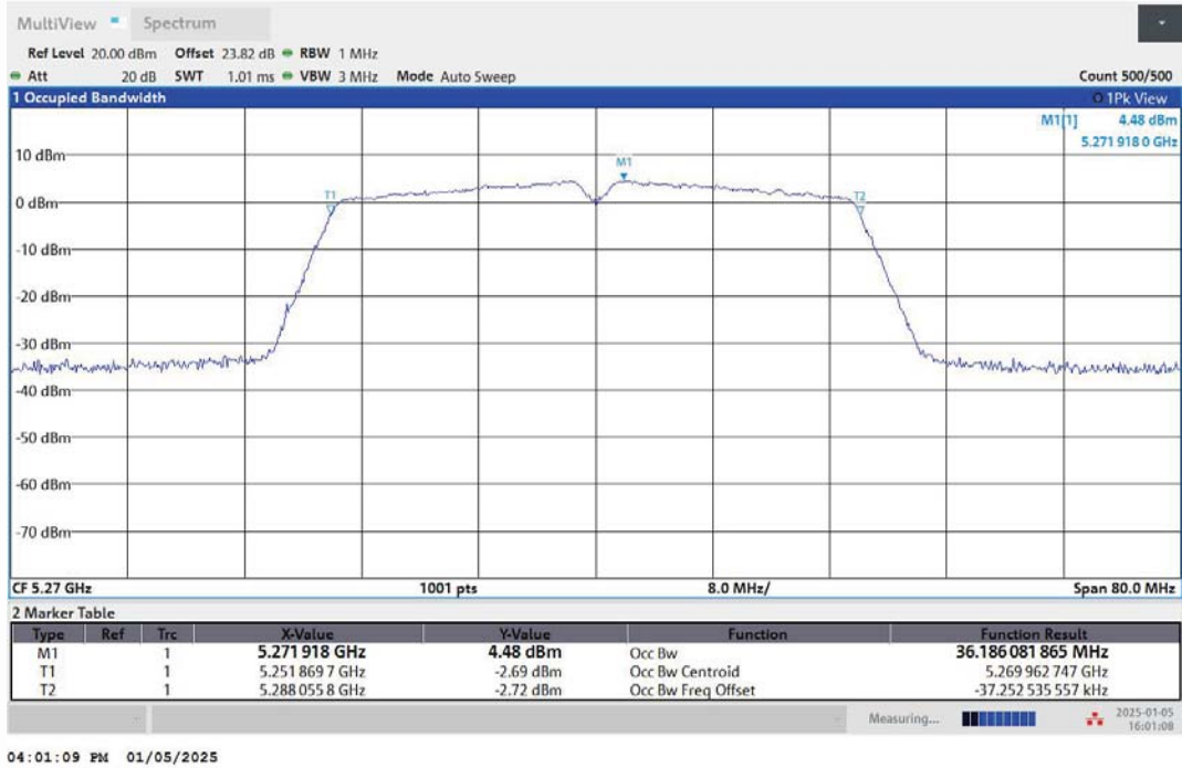
11N40MIMO-Ant1-5270
