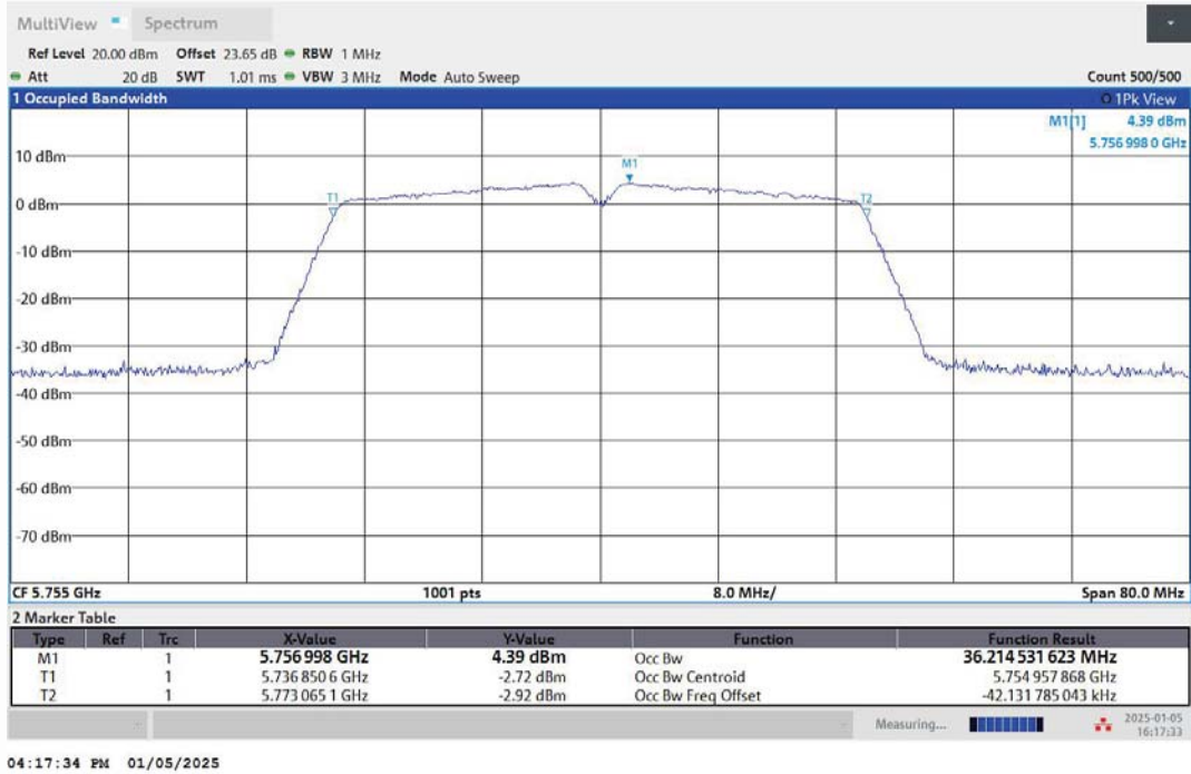
11N40MIMO-Ant1-5755
