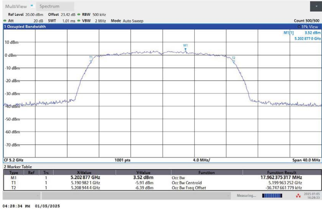
11AC20MIMO-Ant1-5200
