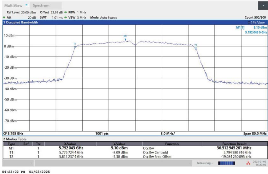
11N40MIMO-Ant2-5795
