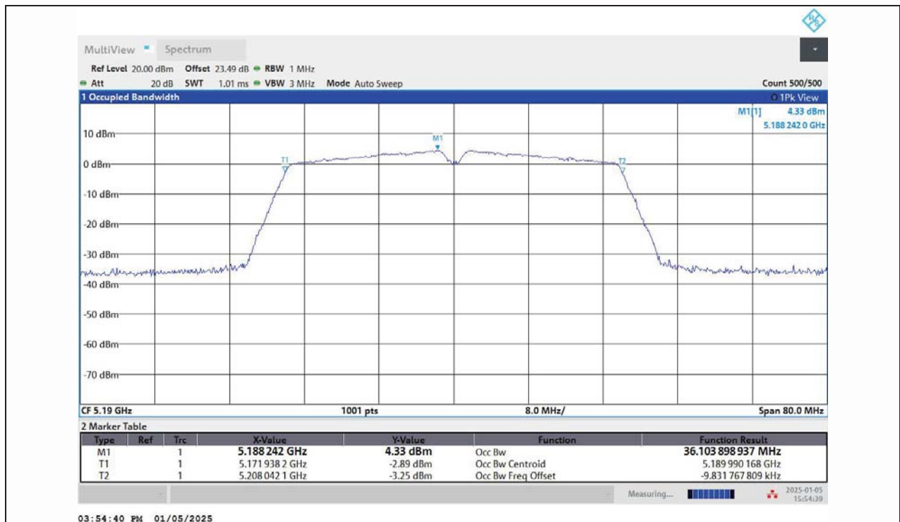
11N40MIMO-Ant1-5190
