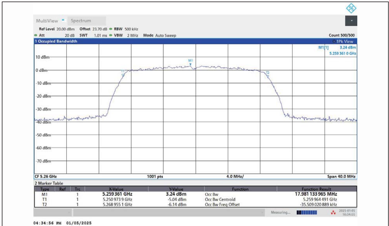
11AC20MIMO-Ant1-5260
