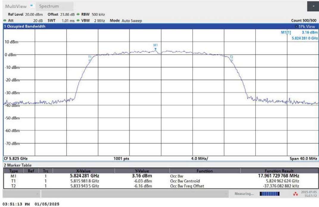
11N20MIMO-Ant1-5825
