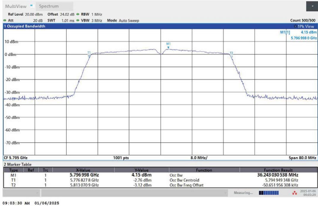
11AC40MIMO-Ant1-5795
