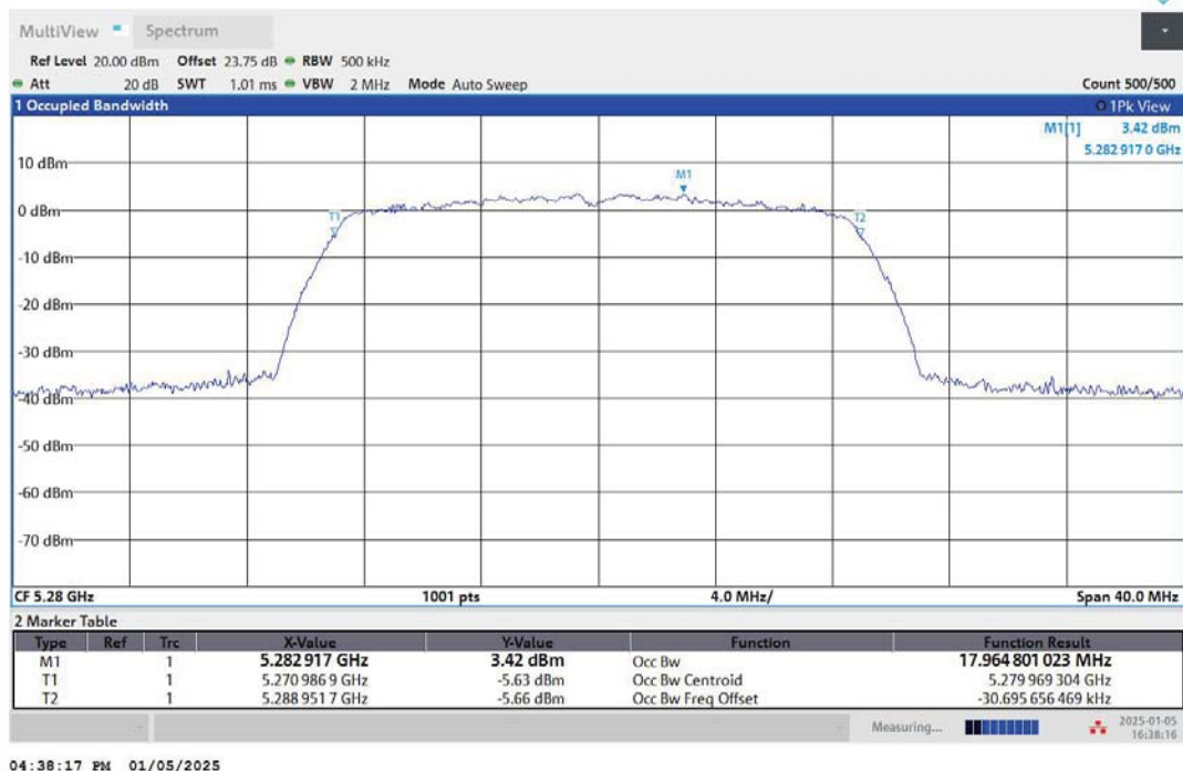
11AC20MIMO-Ant1-5280
