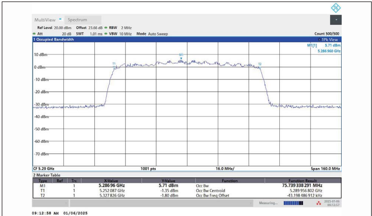
11AC80MIMO-Ant1-5290
