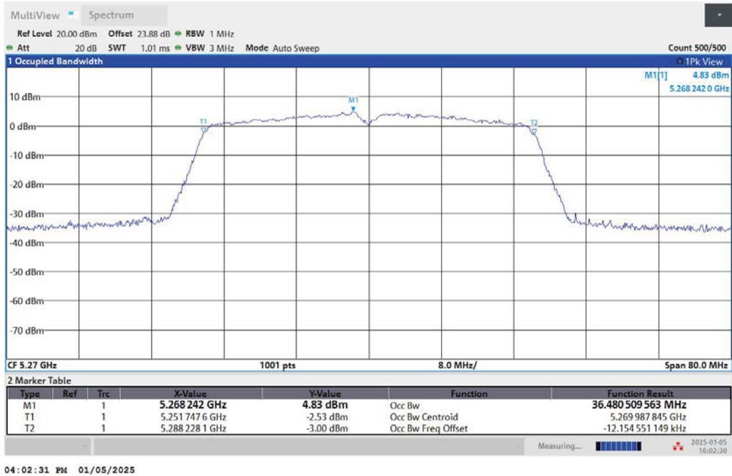
11N40MIMO-Ant2-5270
