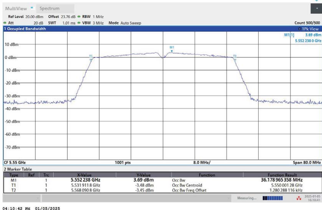
11N40MIMO-Ant1-5550
