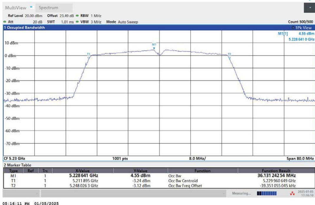
11AC40MIMO-Ant1-5230
