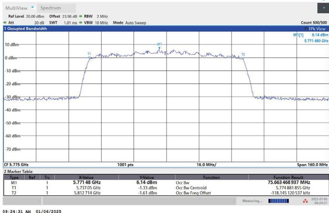
11AC80MIMO-Ant1-5775
