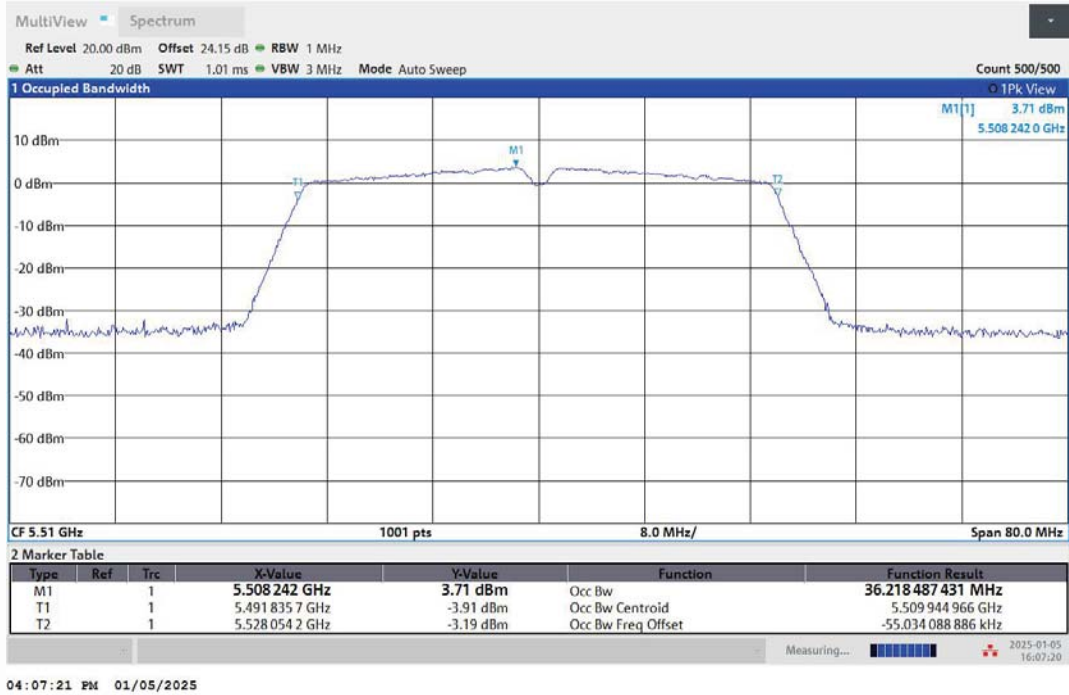
11N40MIMO-Ant1-5510
