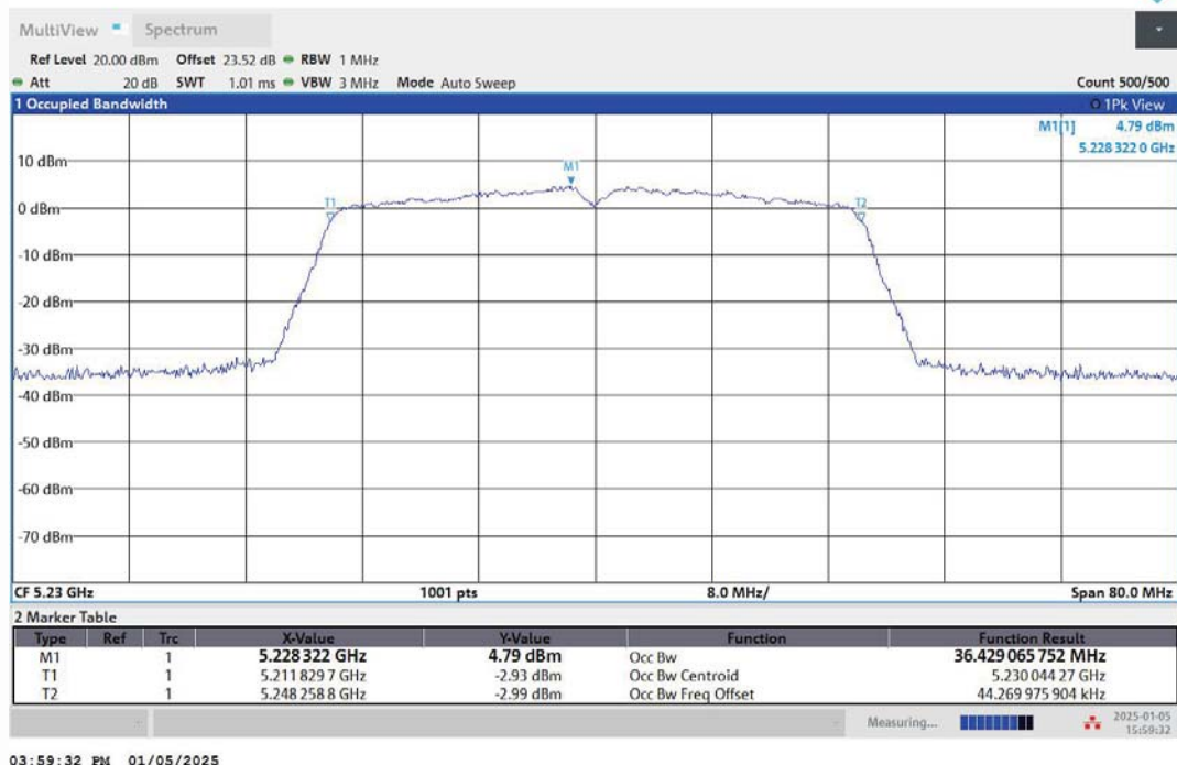
11N40MIMO-Ant2-5230
