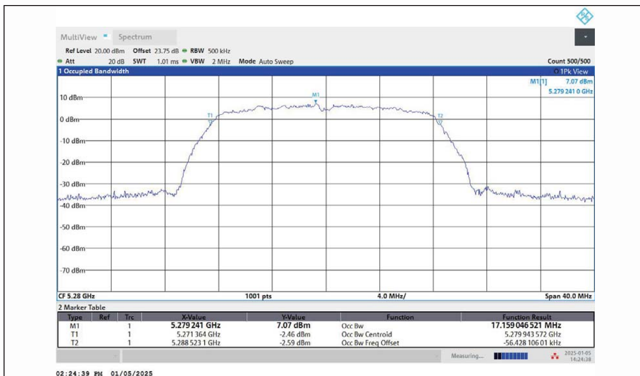
11A-Ant1-5280
