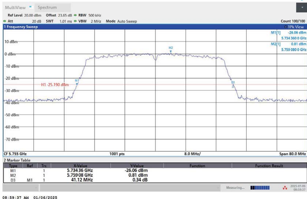
11AC40MIMO-Ant1-5755
