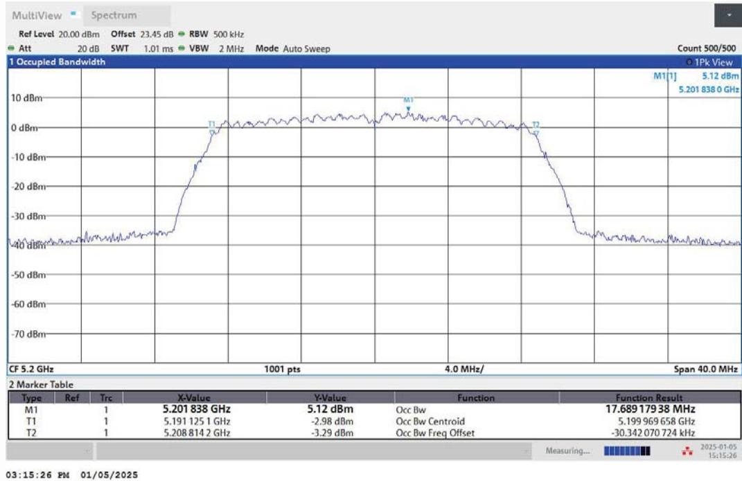
11N20MIMO-Ant2-5200
