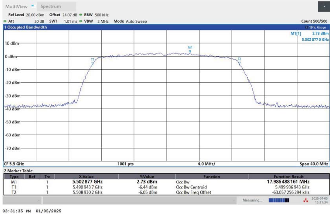
11N20MIMO-Ant1-5500
