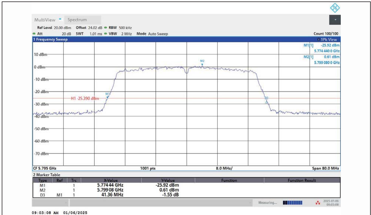
11AC40MIMO-Ant1-5795
