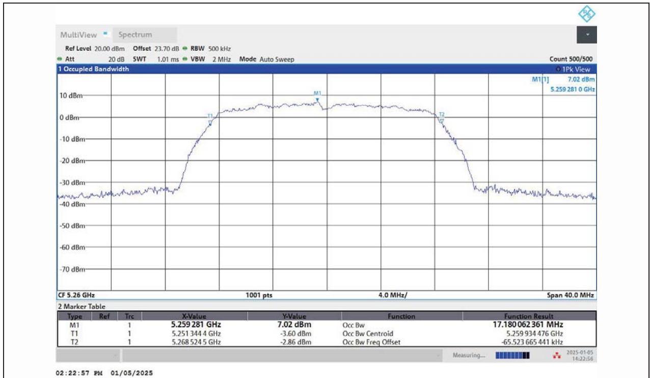
11A-Ant1-5260
