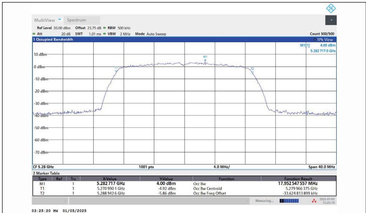
11N20MIMO-Ant1-5280
