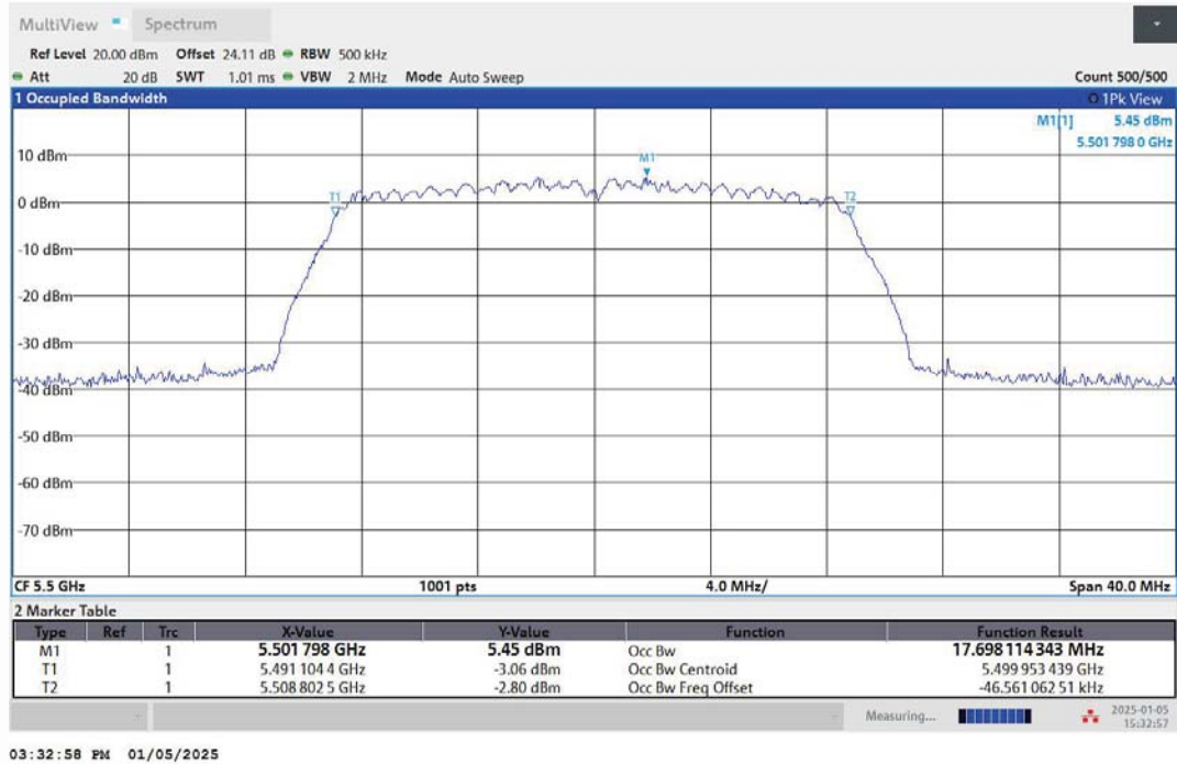
11N20MIMO-Ant2-5500
