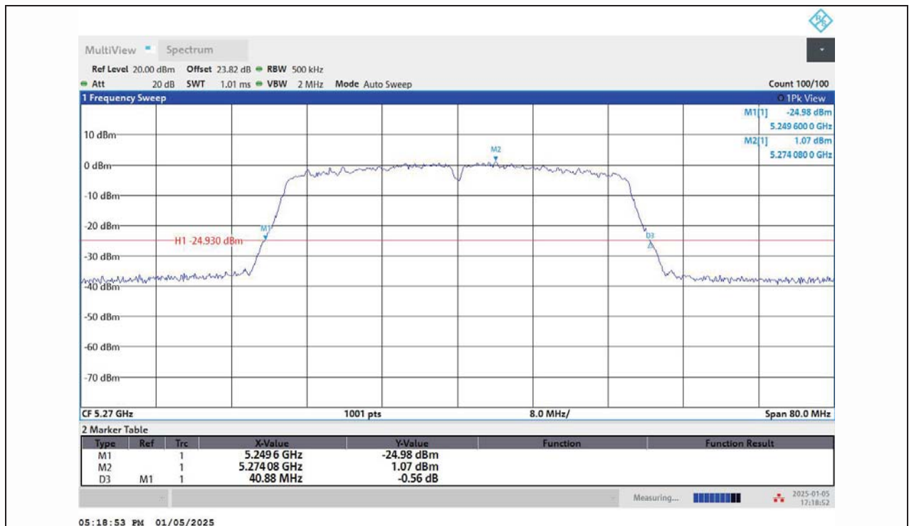
11AC40MIMO-Ant1-5270
