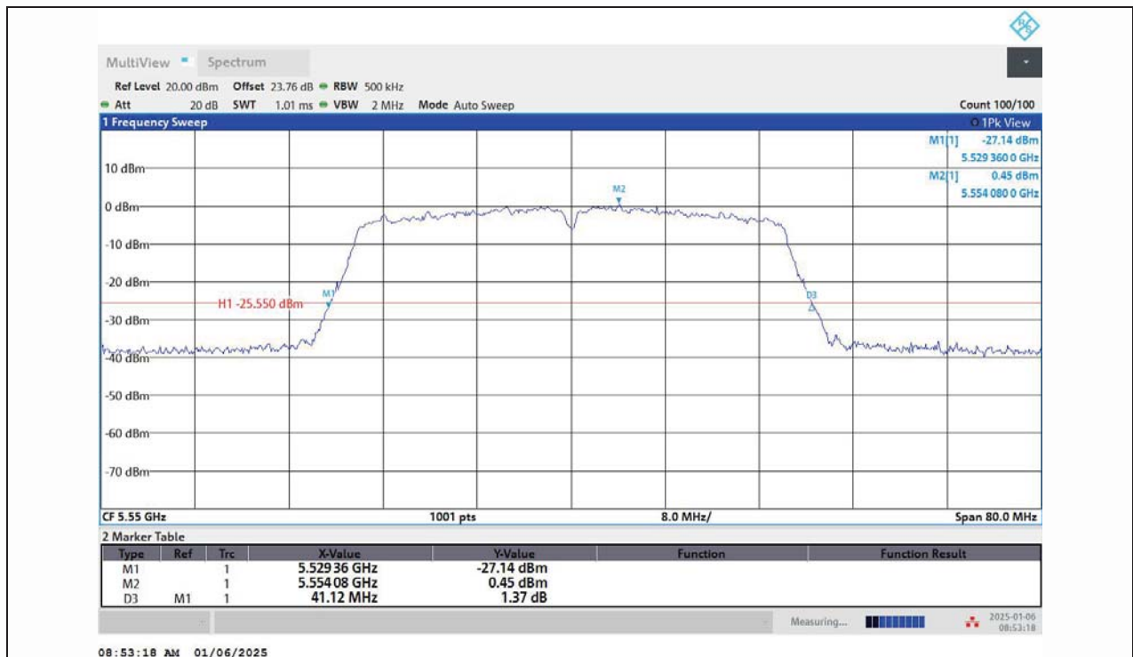
11AC40MIMO-Ant1-5550
