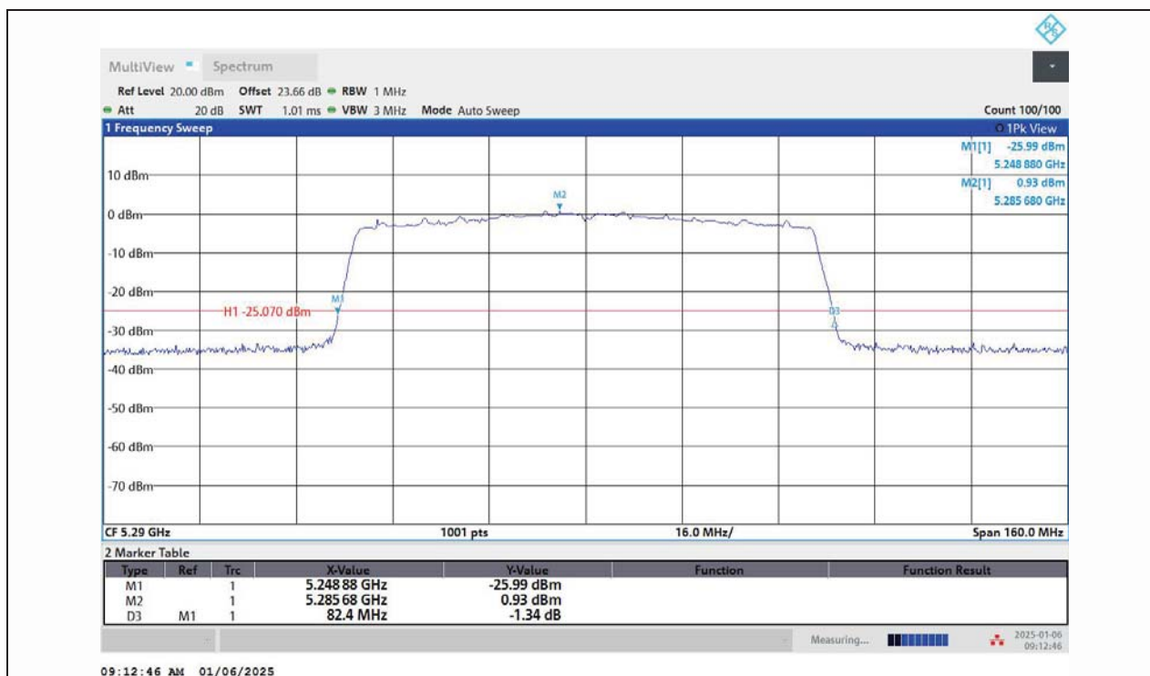
11AC80MIMO-Ant1-5290
