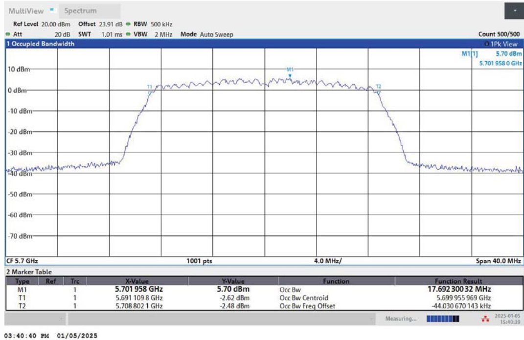
11N20MIMO-Ant2-5700
