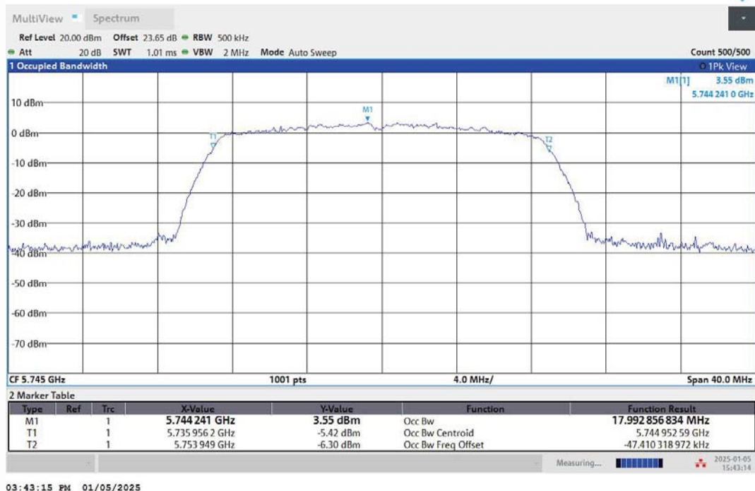
11N20MIMO-Ant1-5745
