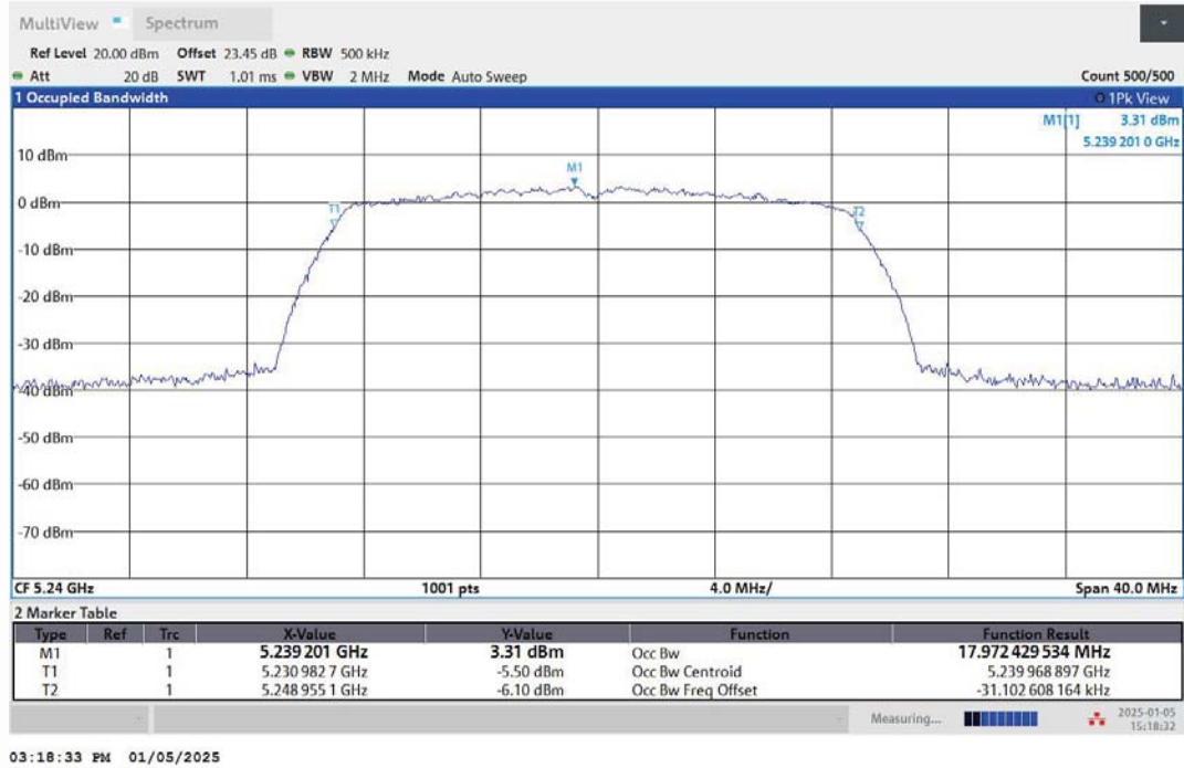
11N20MIMO-Ant1-5240
