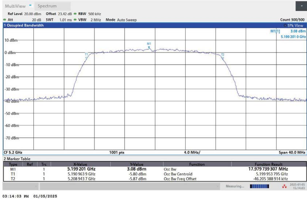
11N20MIMO-Ant1-5200
