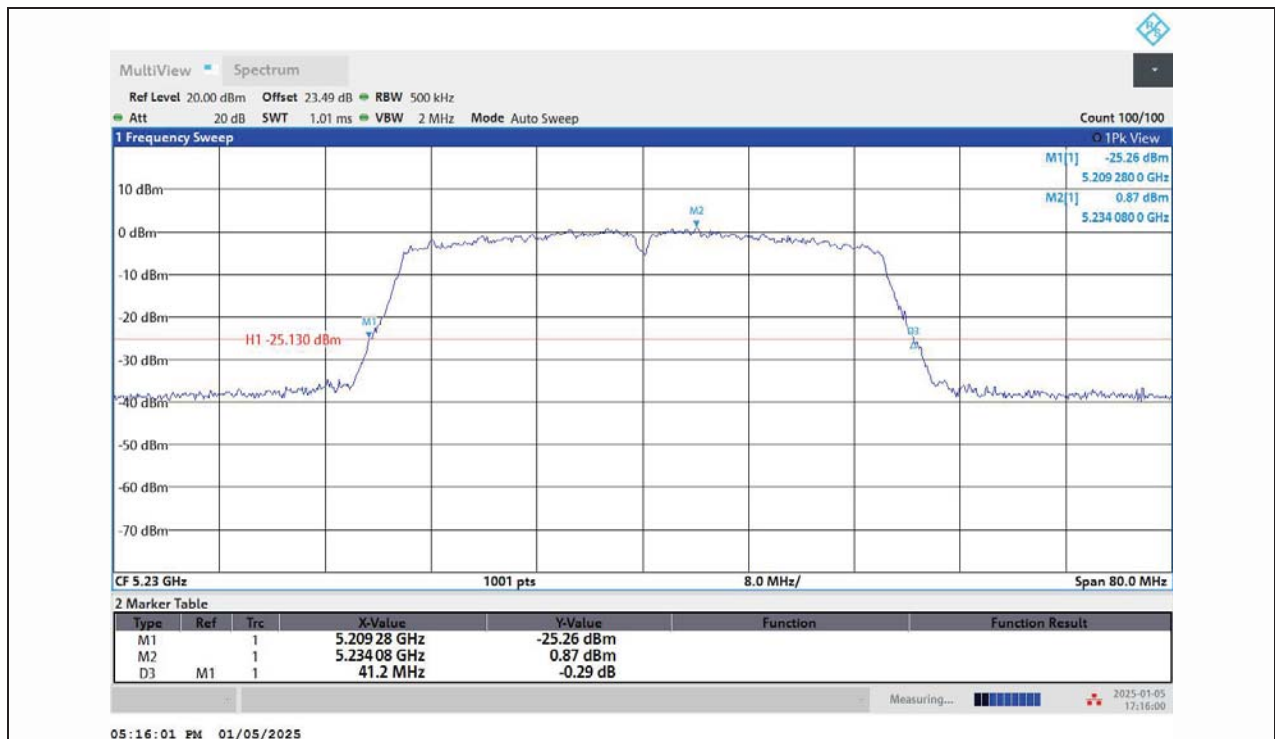
11AC40MIMO-Ant1-5230
