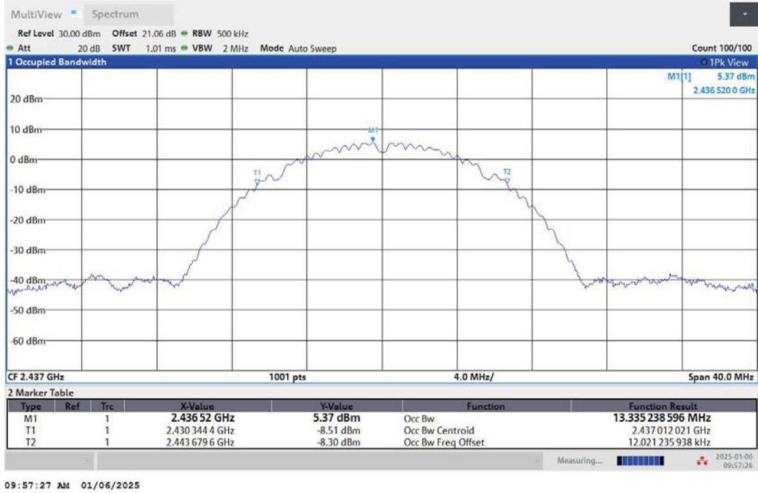
11B-Ant1-2437
