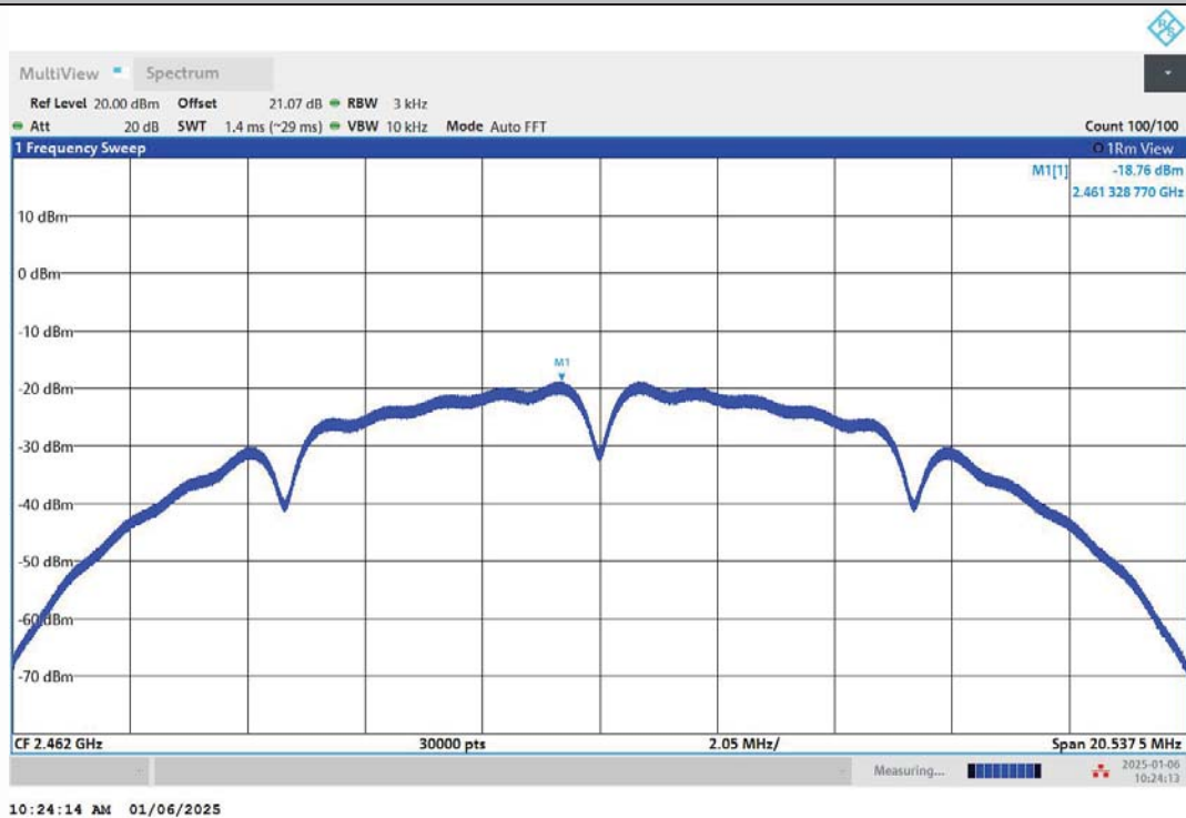
11B-Ant2-2462-PASS
