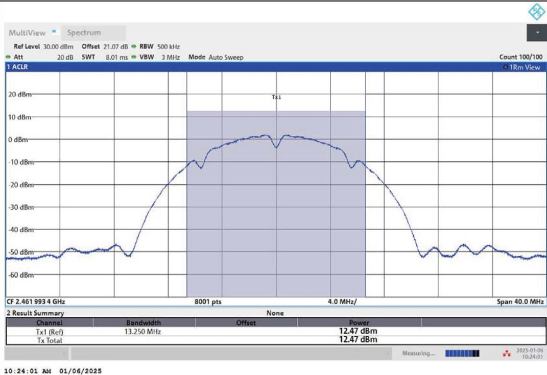
11B-Ant2-2462-PASS
