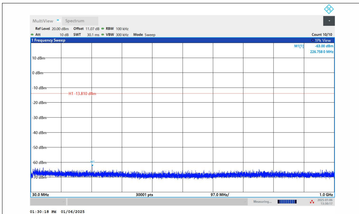
BLE_2M-Ant1-2440-30~1000-PASS
