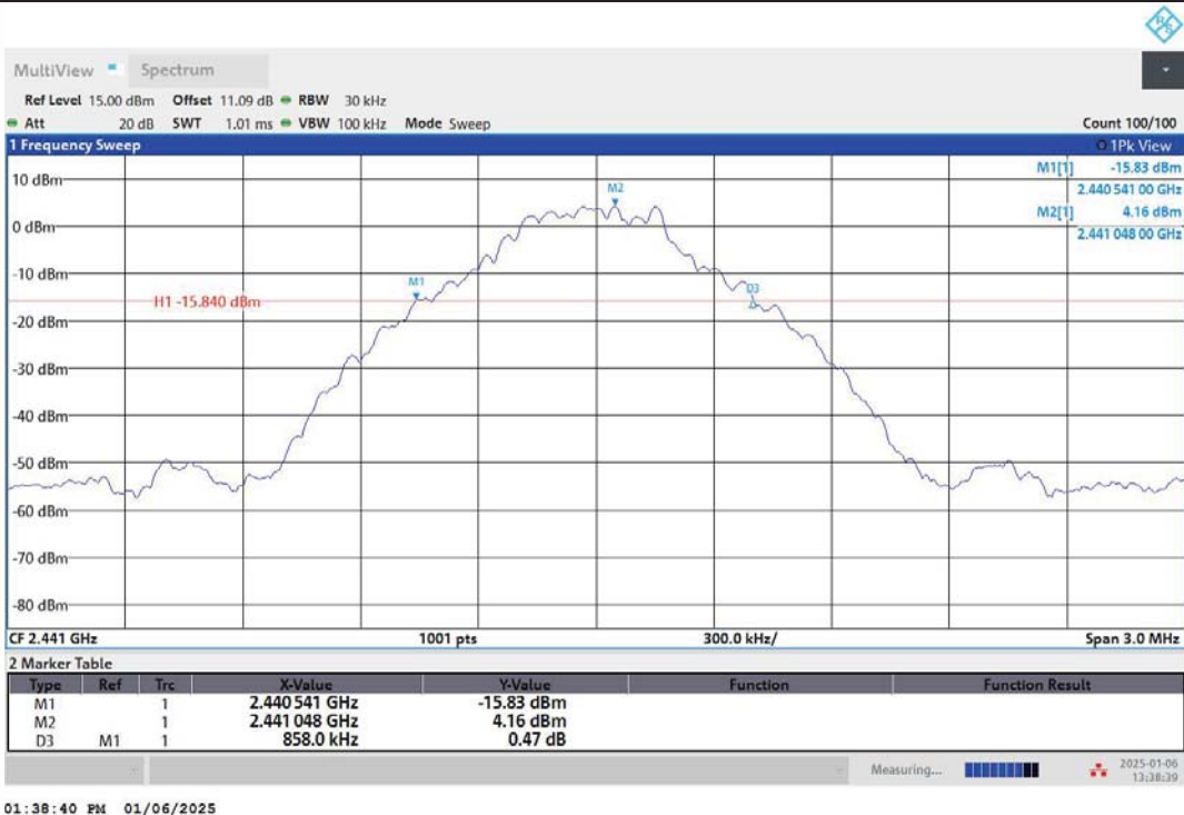
DH5-Ant1-2441
