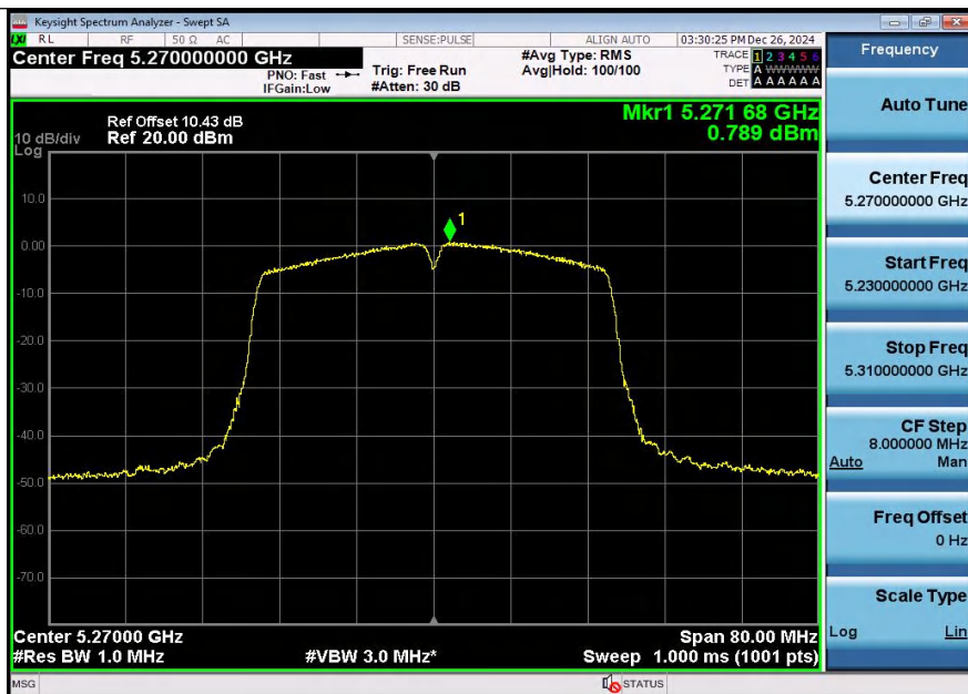
11N40SISO-Ant2-5270-PASS
