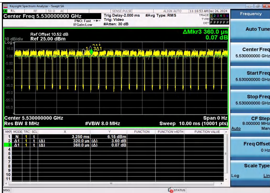
NTNV-11AC80SISO-Ant1-5530
