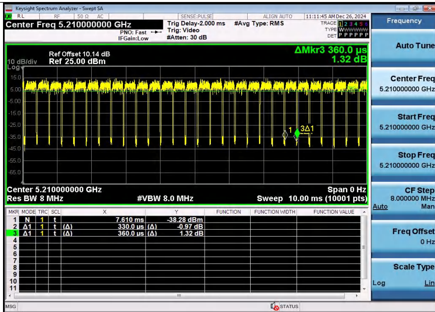
NTNV-11AC80SISO-Ant1-5210
