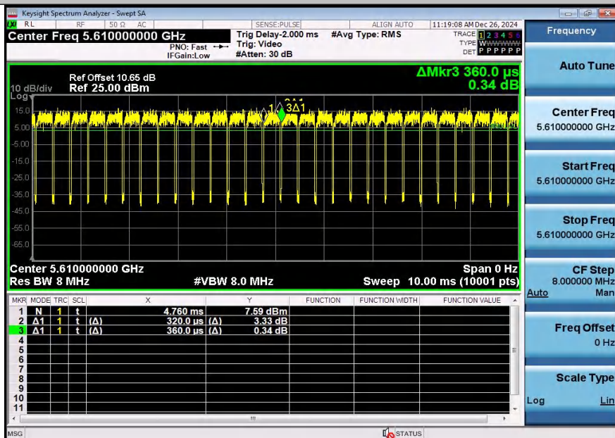
NTNV-11AC80SISO-Ant1-5610
