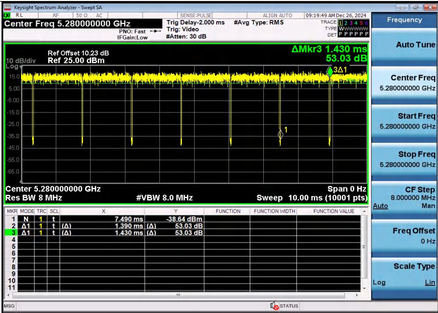
NTNV-11A-Ant1-5280
