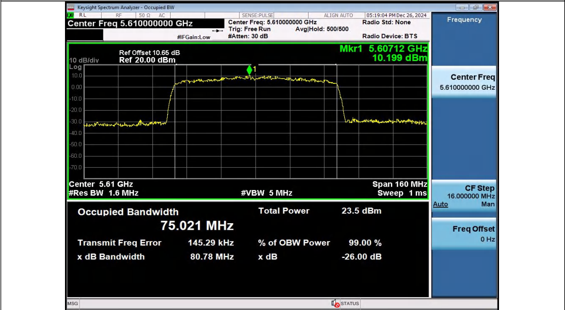
11AC80SISO-Ant2-5610
