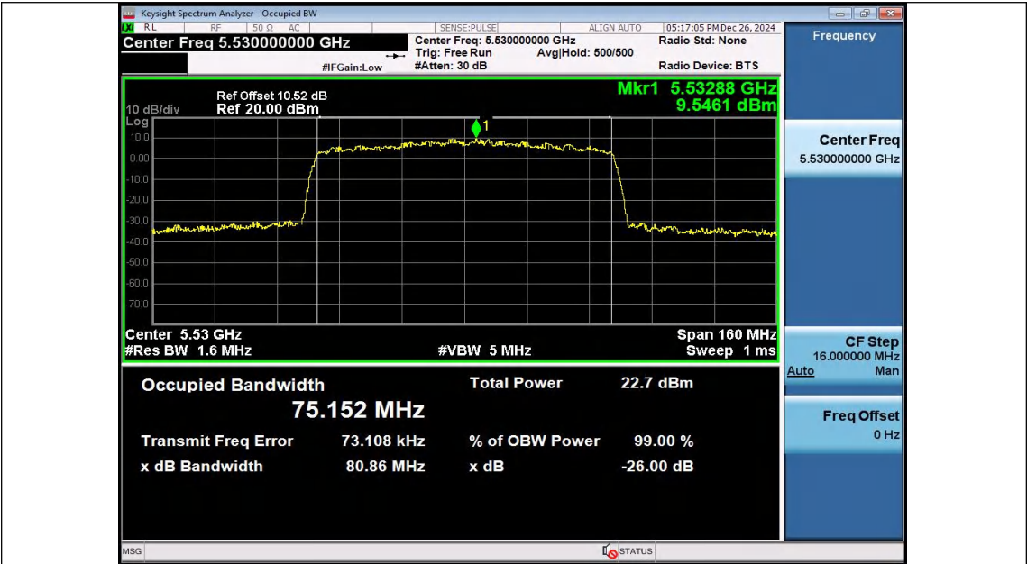
11AC80SISO-Ant2-5530
