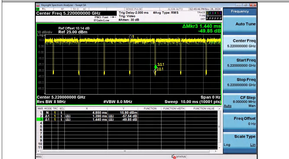
NTNV-11A-Ant2-5220
