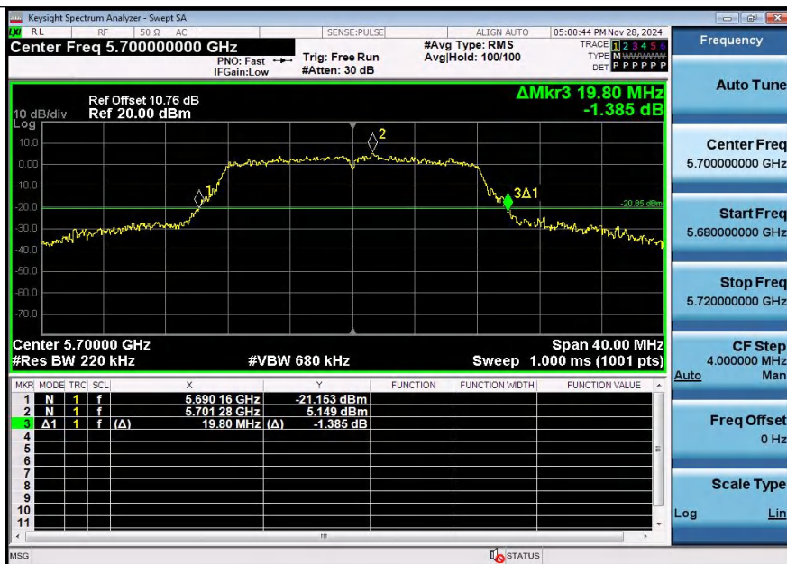
11A-Ant1-5700
