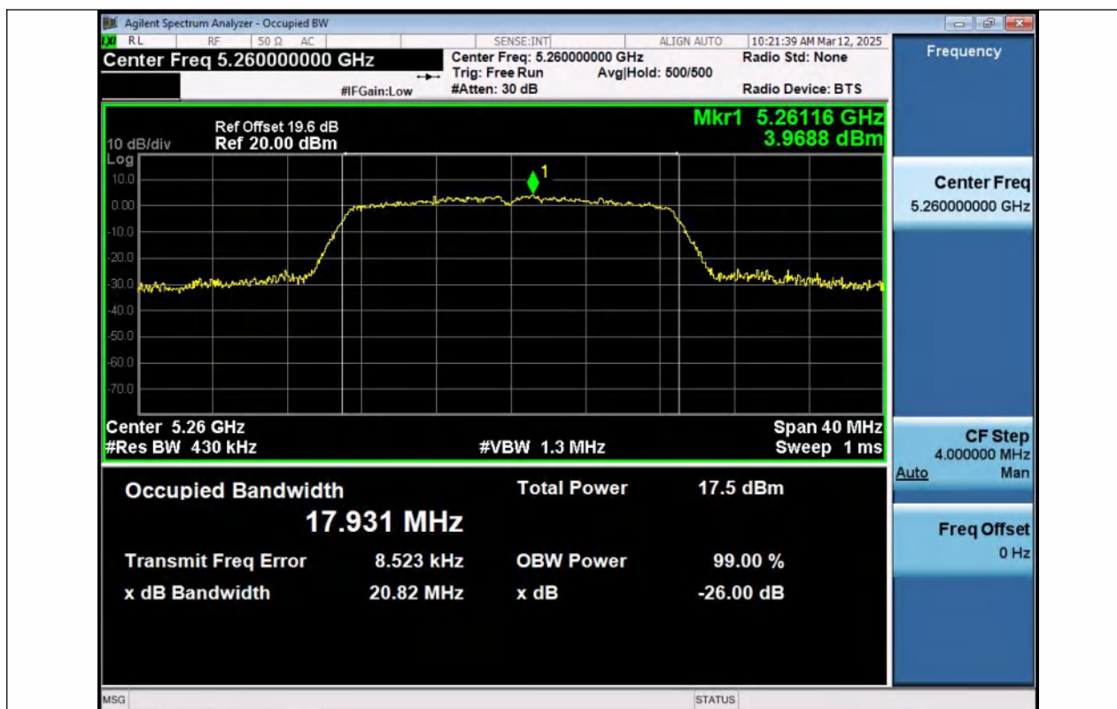
11AC20MIMO-Ant1-5260
