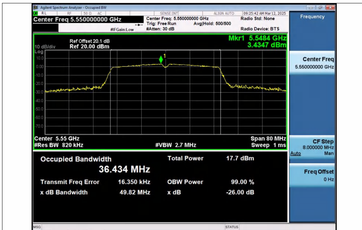
11N40MIMO-Ant1-5550
