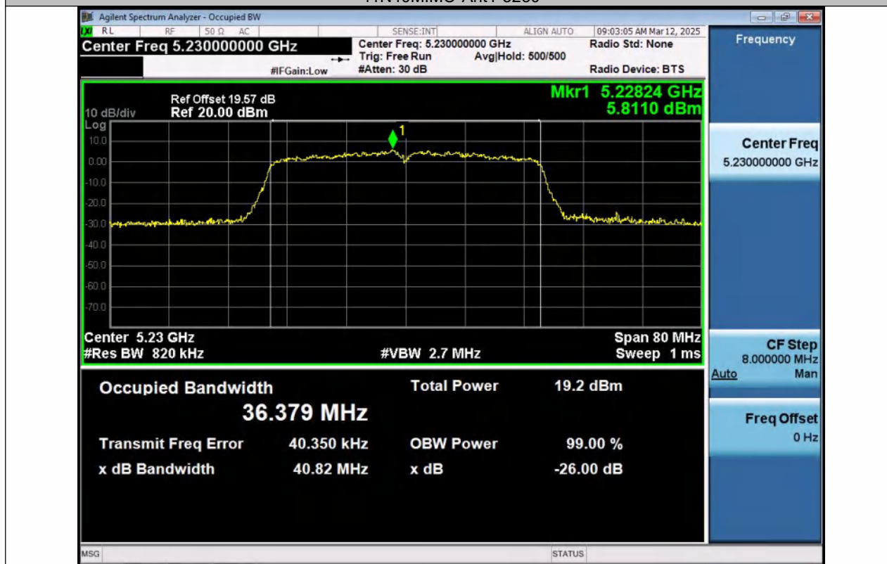
11N40MIMO-Ant2-5230
