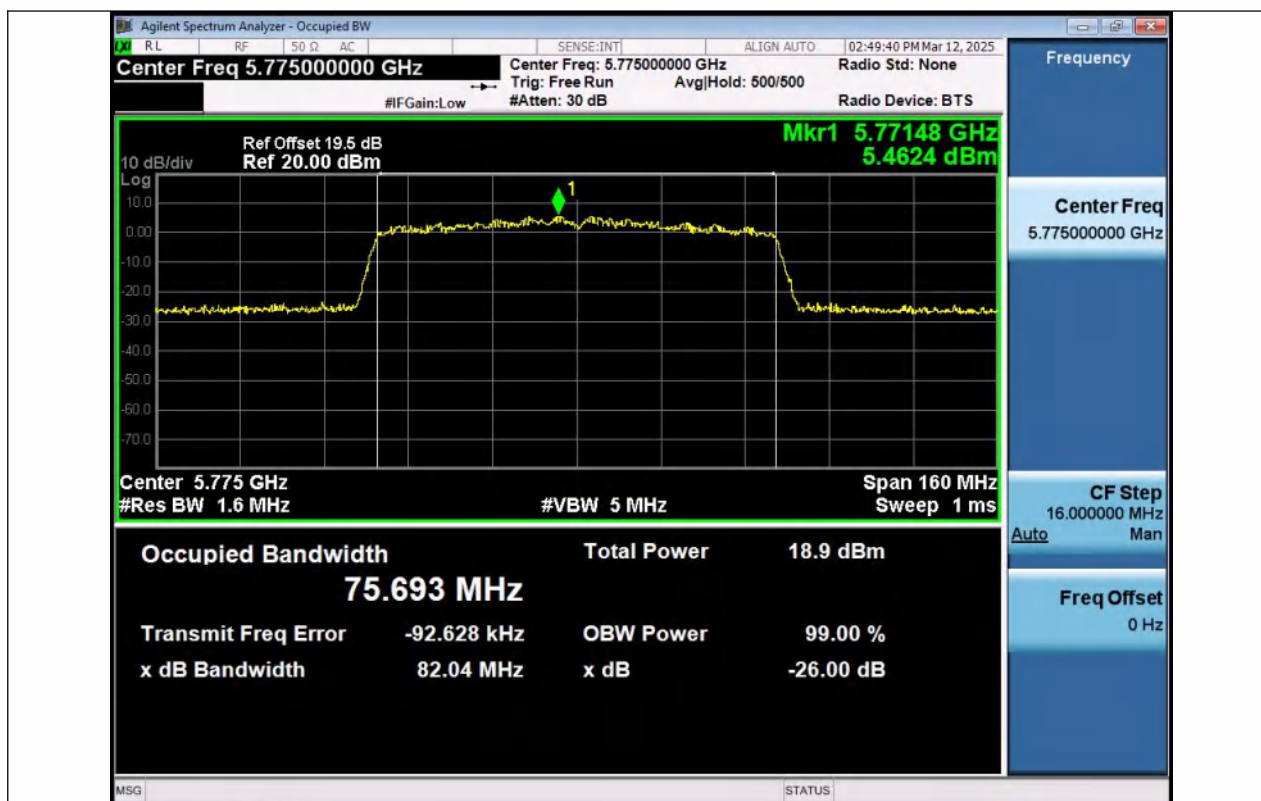
11AC80MIMO-Ant1-5775
