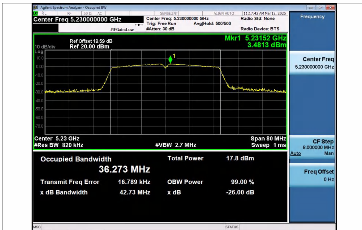
11AC40MIMO-Ant1-5230
