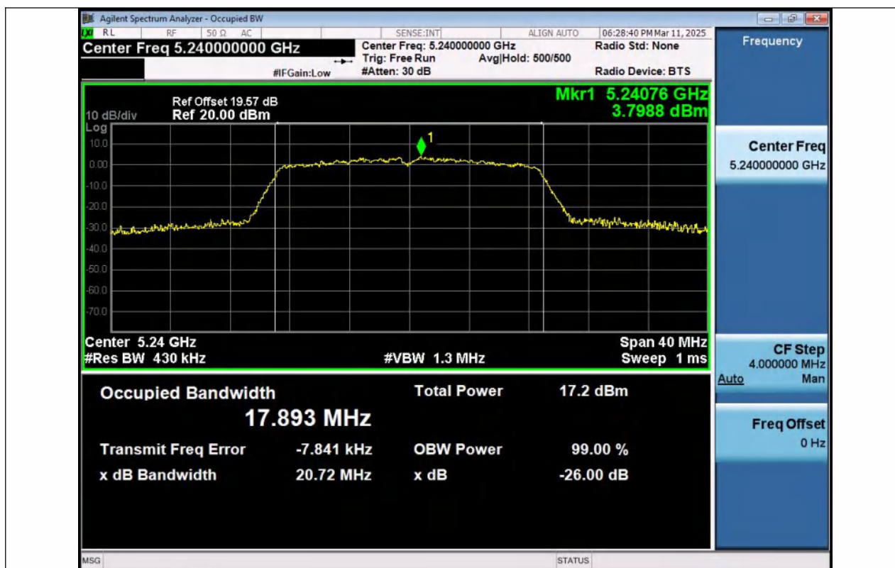
11N20MIMO-Ant1-5240
