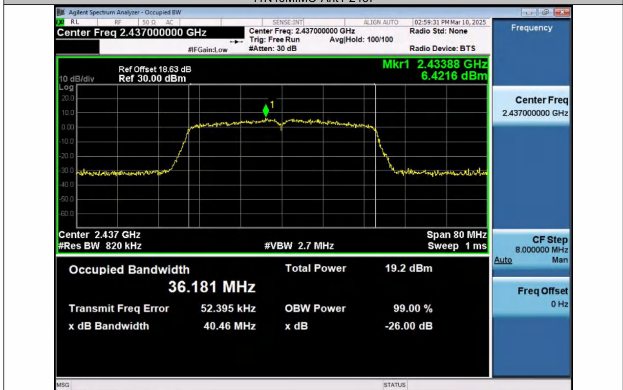
11N40MIMO-Ant2-2437
