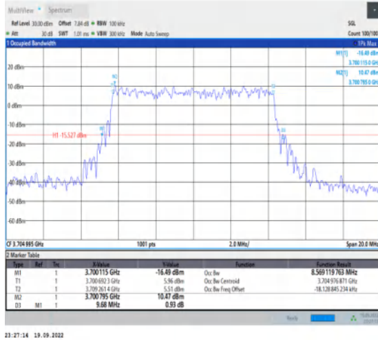
1-N78-3700-3800-30-10-L-5-DFT-256QAM-Outet_Fu II-24@0-Ant1-8.569-9.680-≤10-PASS
