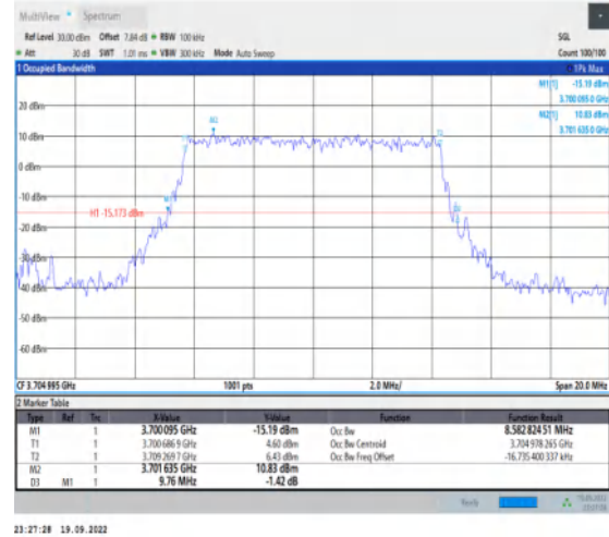
1-N78-3700-3800-30-10-L-6-CP-QPSK-Outet_Full-2 4@0-Ant1-8.583-9.760-≤10-PASS
