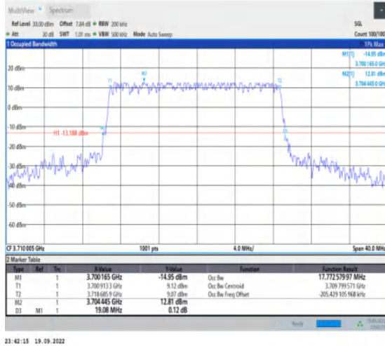
1-N78-3700-3800-30-20-L-3-DFT-16QAM-Outer_Full -50@0-Ant1-17.773-19.080-≤20-PASS
