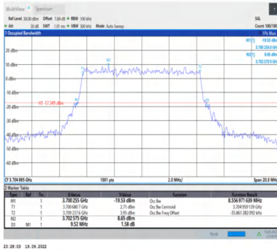
1-N78-3700-3800-30-10-L-9-CP-256QAM-Outer_Full -24@0-Ant1-8.557-9.520-≤10-PASS
