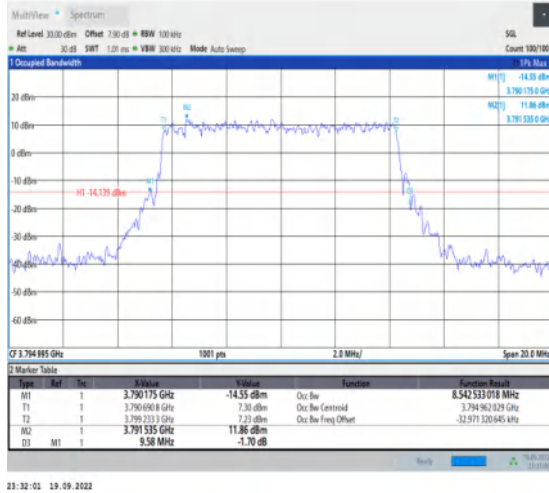
1-N78-3700-3800-30-10-H-3-DFT-16QAM-Outer_Ful I-24@0-Ant1-8.543-9.580-≤10-PASS
