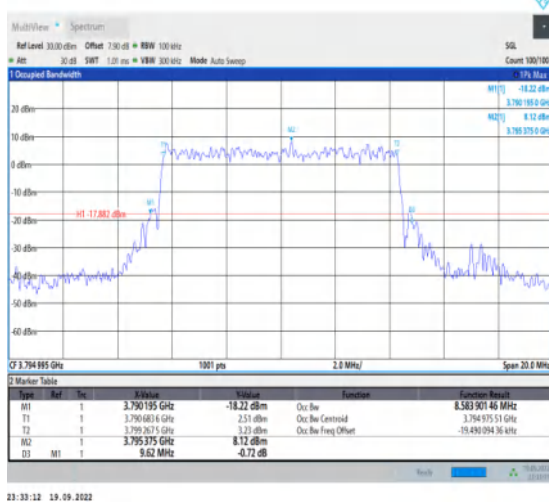
1-N78-3700-3800-30-10-H-9-CP-256QAM-Outer_Ful-I-24@0-Ant1-8.584-9.620-≤10-PASS
