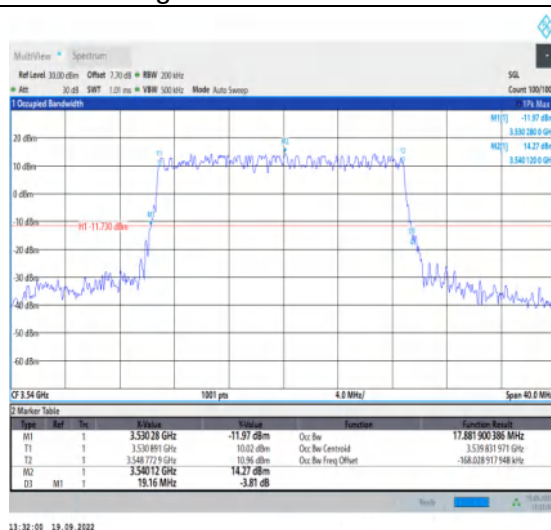
1-N78-3450-3550--30-20-H-2-DFT-PI2BPSK-Outer_Full -50@0-Ant1-17.882-19.160-≤20-PASS
