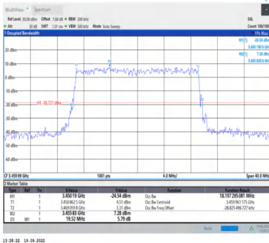
1-N78-3450-3550--30-20-L-9-CP-256QAM-Outer_Fu II-51@0-Ant1-18.197-19.520-≤20-PASS
