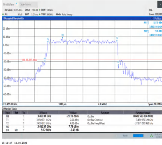
1-N78-3450-3550--30-10-L-9-CP-256QAM-Outer_Fu ll-24@0-Ant1-8.603-9.120-≤10-PASS
