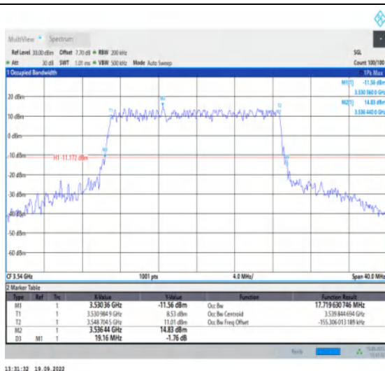
1-N78-3450-3550--30-20-H-1-DFT-QPSK-Outer_Full -50@0-Ant1-17.72-19.160-≤20-PASS
