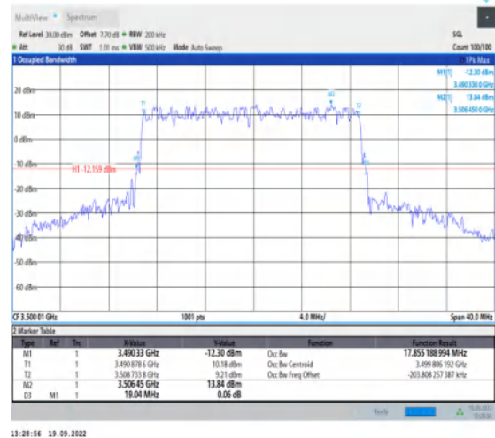
1-N78-3450-3550--30-20-M-1-DFT-QPSK-Outer_Full -50@0-Ant1-17.855-19.040-≤20-PASS
