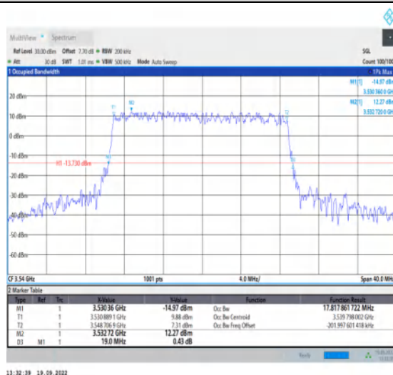
1-N78-3450-3550--30-20-H-4-DFT-64QAM-Outer_Fu II-50@0-Ant1-17.818-19.000-≤20-PASS
