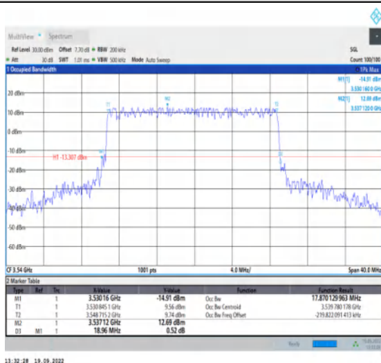
1-N78-3450-3550--30-20-H-3-DFT-16QAM-Outer_Fu II-50@0-Ant1-17.87-18.960-≤20-PASS
