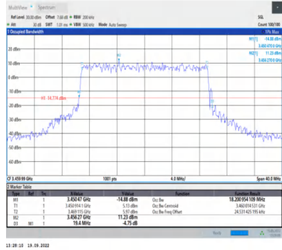
1-N78-3450-3550--30-20-L-8-CP-64QAM-Outer_Full -51@0-Ant1-18.201-19.400-≤20-PASS
