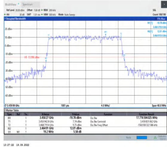
1-N78-3450-3550--30-20-L-4-DFT-64QAM-Outer_Ful l-50@0-Ant1-17.777-19.200-<20-PASS
