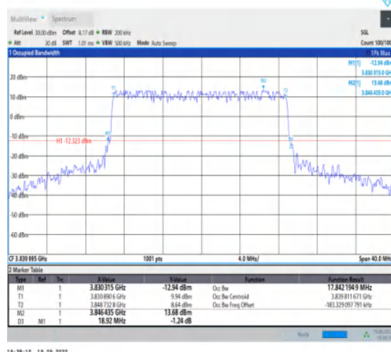
1-N77-3700-3980--30-20-M-1-DFT-QPSK-Outer_Full -50@0-Ant1-17.842-18.920-≤20-PASS
