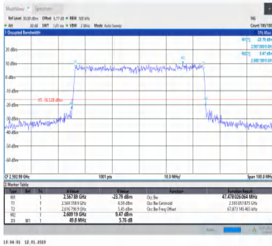
1-N41-PC3-30-50-M-7-CP-16QAM-Outer_Full-133@ 0-Ant1-47.478-49.800-≤50-PASS
