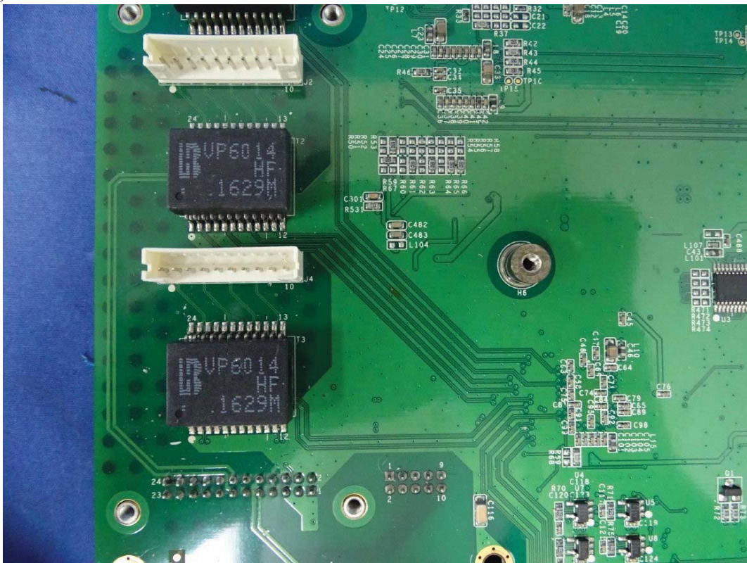
(44) EUT Photo
