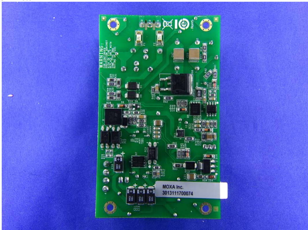
(44) EUT Photo
