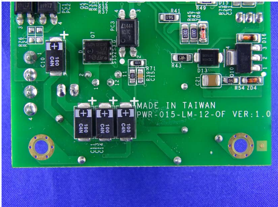
(48) EUT Photo
