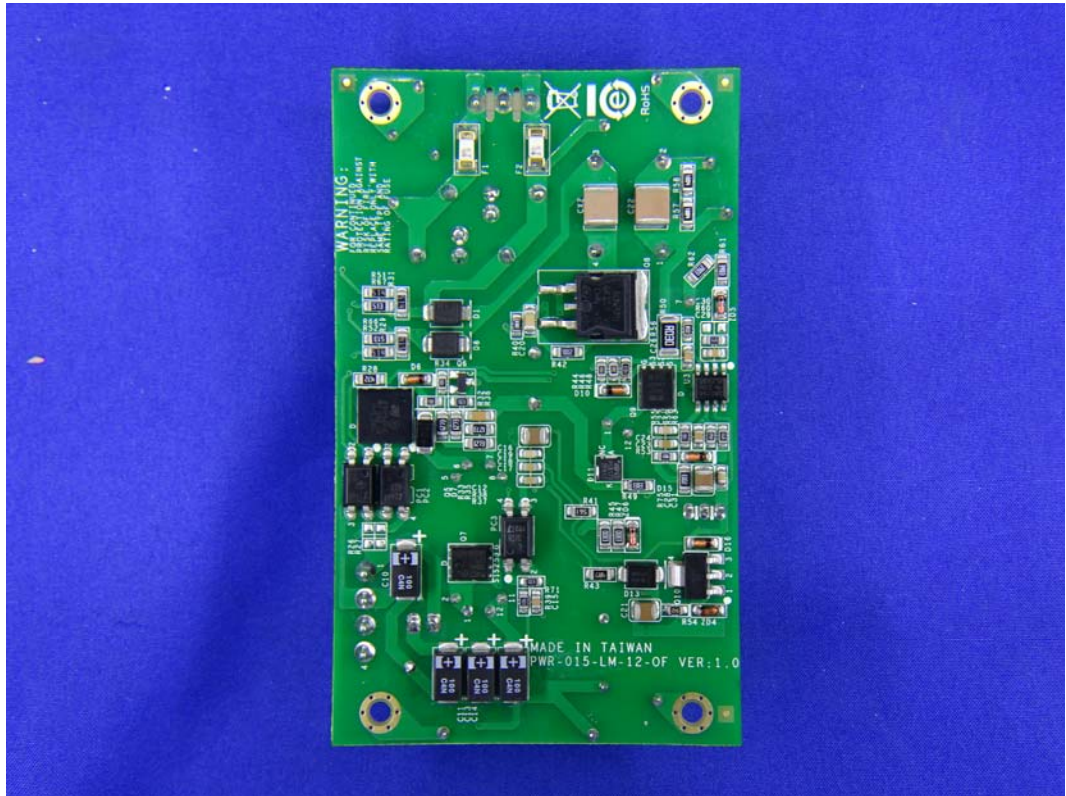
(46) EUT Photo
