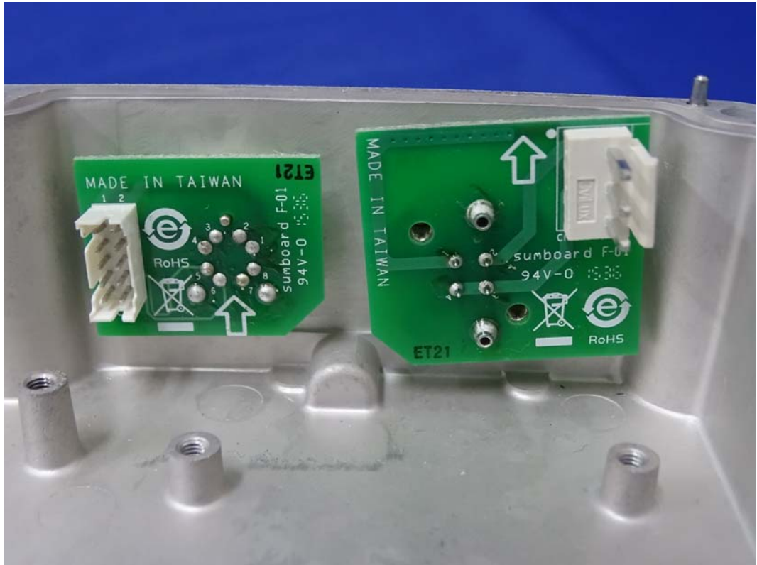
(52) EUT Photo
