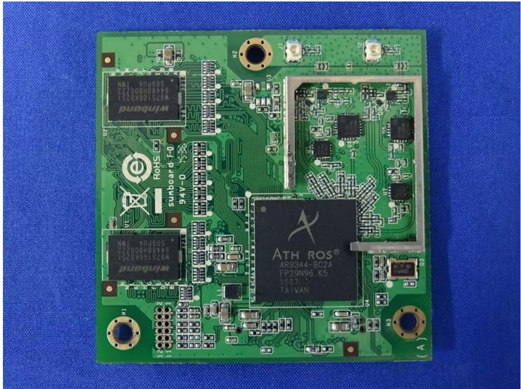
(36) EUT Photo
