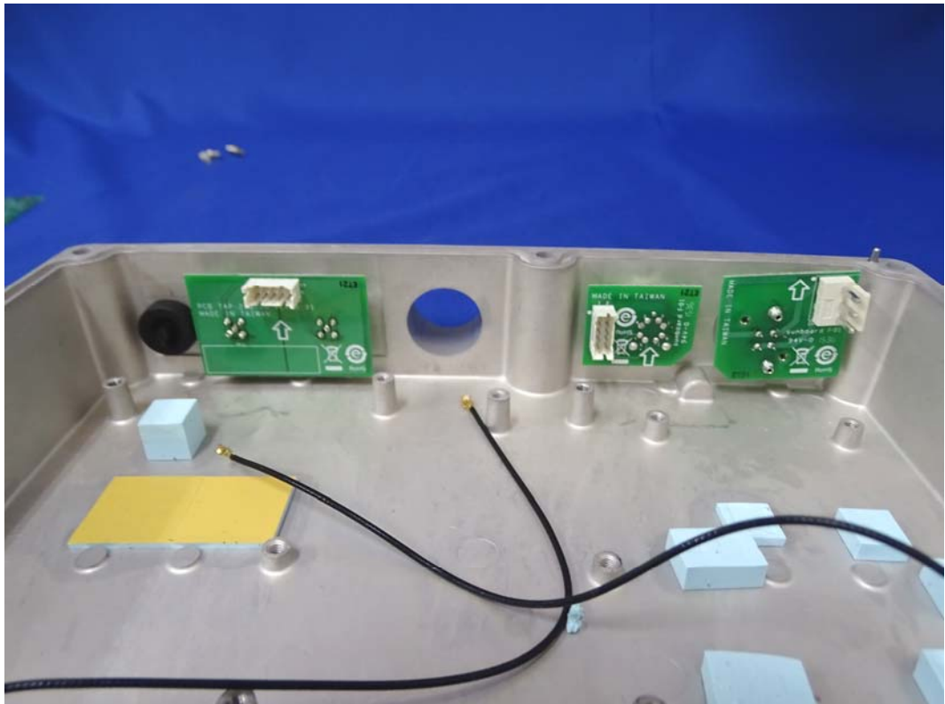
(50) EUT Photo
