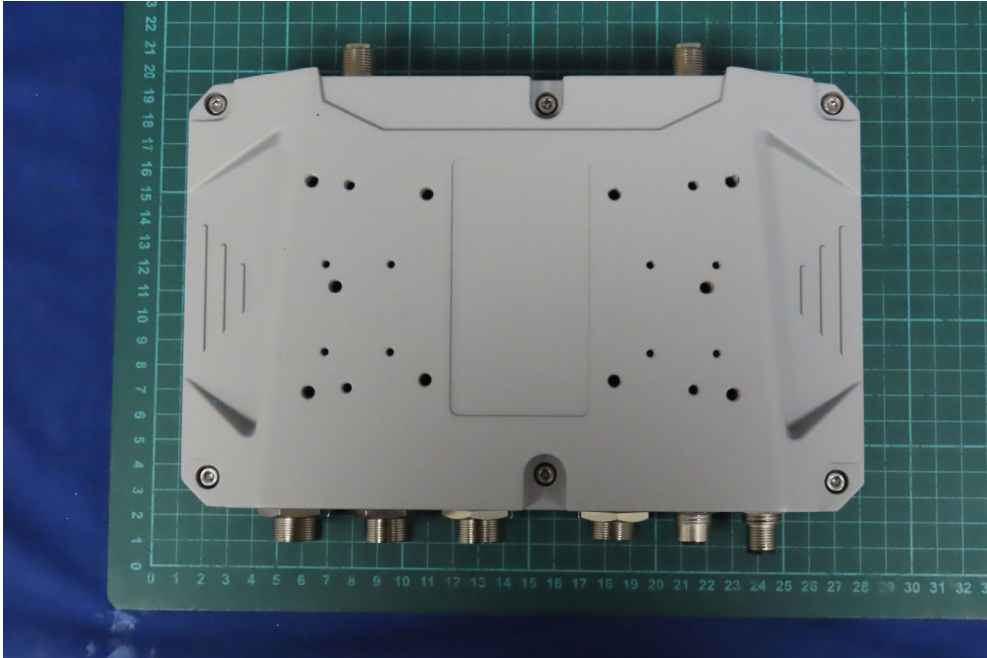
(2) EUT Photo
