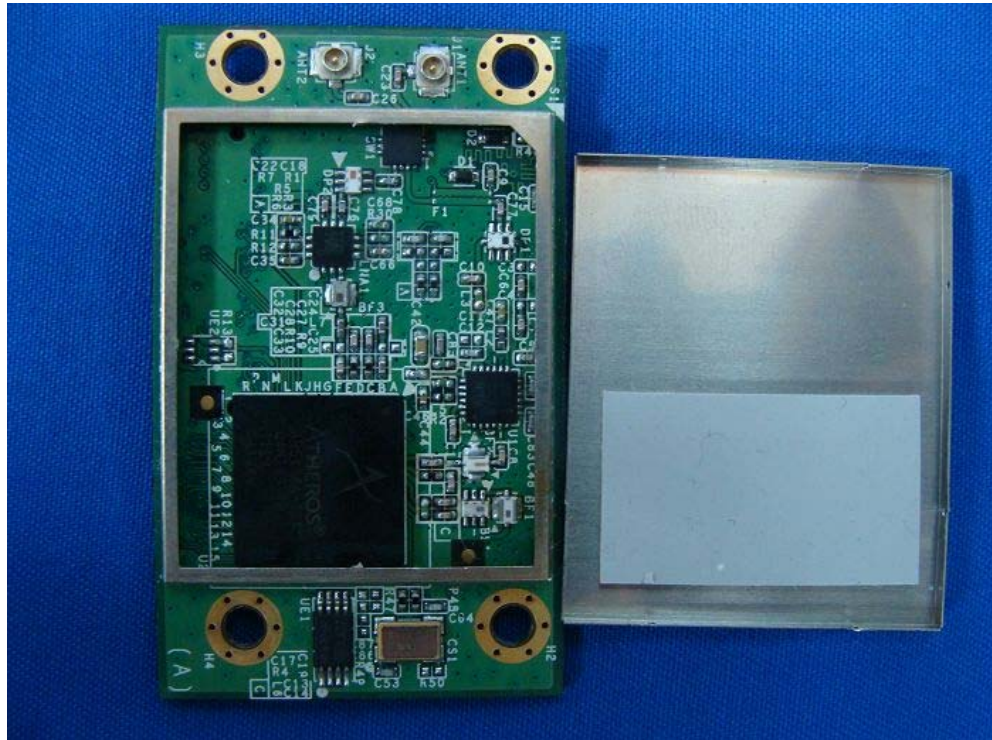
(3) EUT Photo
