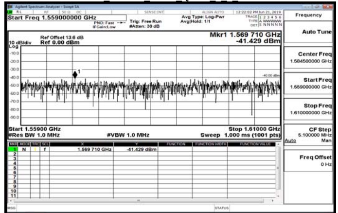
1559MHz~1610MHz Band13 5MHz QPSK 1 0 LowCH23205-779.5
