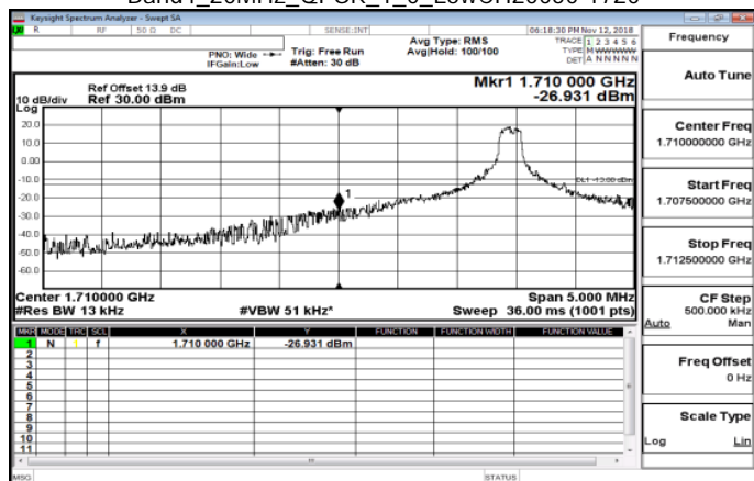
Band4_20MHz_QPSK_1_0_LowCH20050-1720
